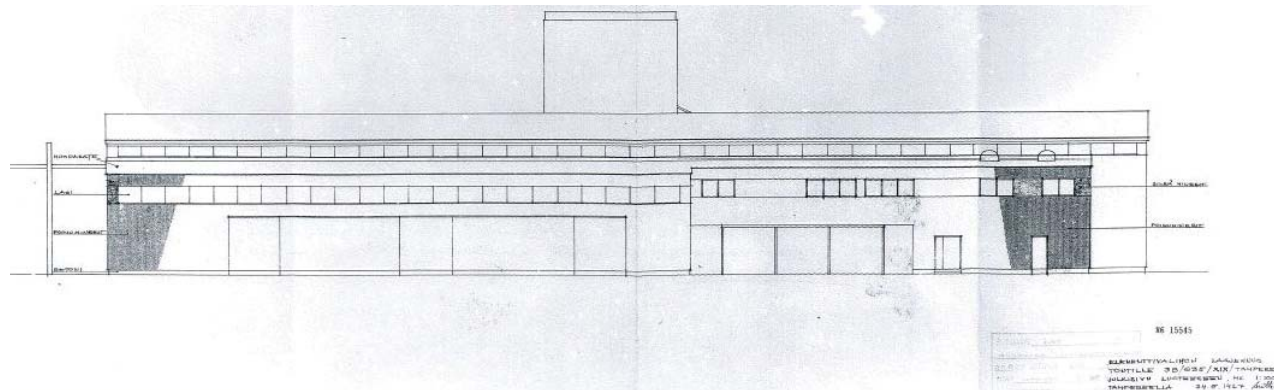
Tampereen Elementti Oy 1967. Olavi Murtomäki ja Stig Lindholm. Tampereen kaupungin rakennusvalvonnan piirustusarkisto. Tampereen kaupungin rakennusvalvonnan piirustusarkisto.
