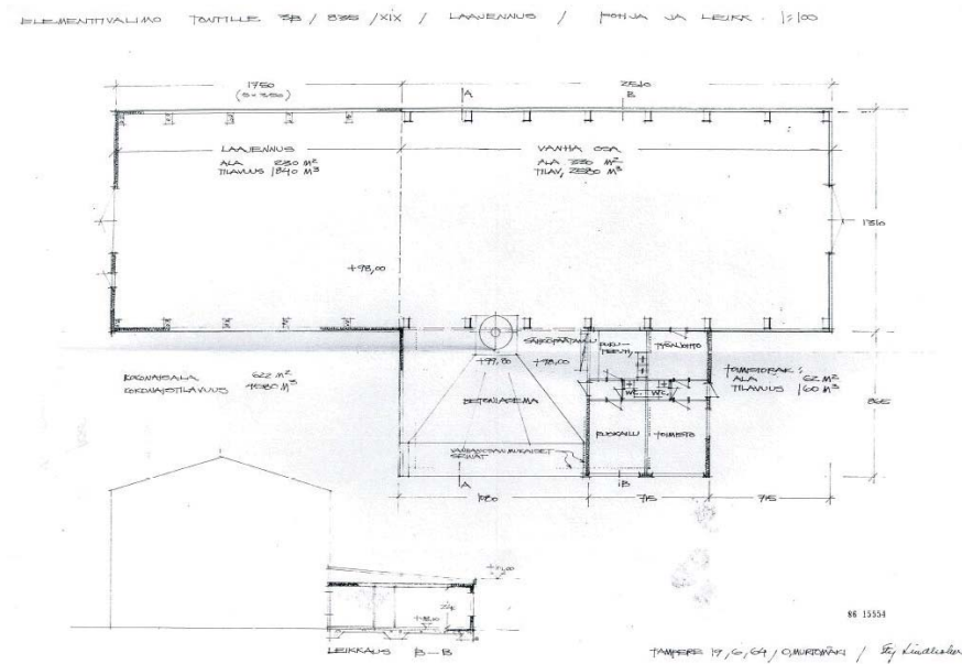
Tampereen Elementti Oy 1964. Olavi Murtomäki ja Stig Lindholm. Tampereen kaupungin rakennusvalvonnan piirustusarkisto. Tampereen kaupungin rakennusvalvonnan piirustusarkisto.
