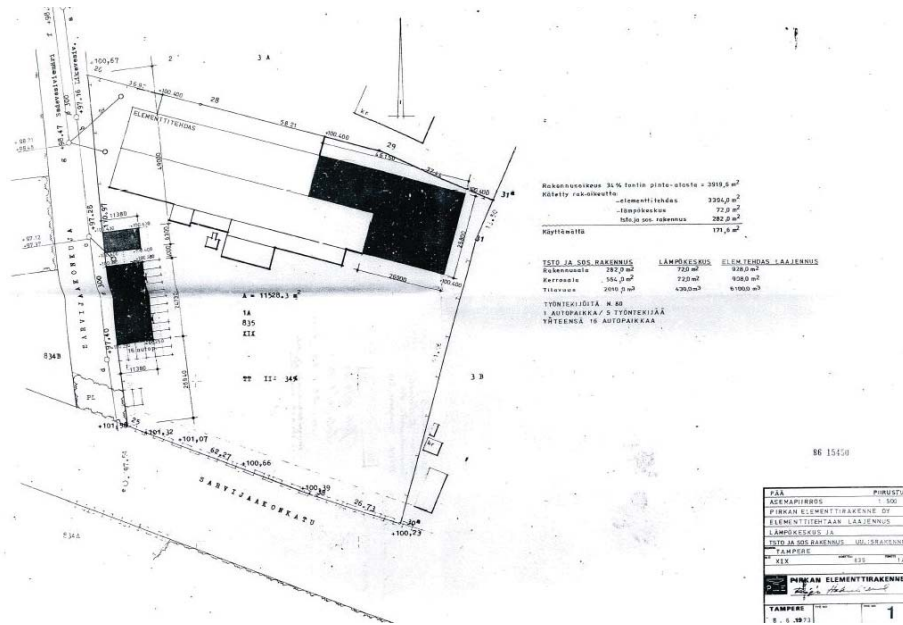
Pirkan Elementtirakenne Oy:n asemapiirros 1973. Tampereen kaupungin rakennusvalvonnan piirustusarkisto.
