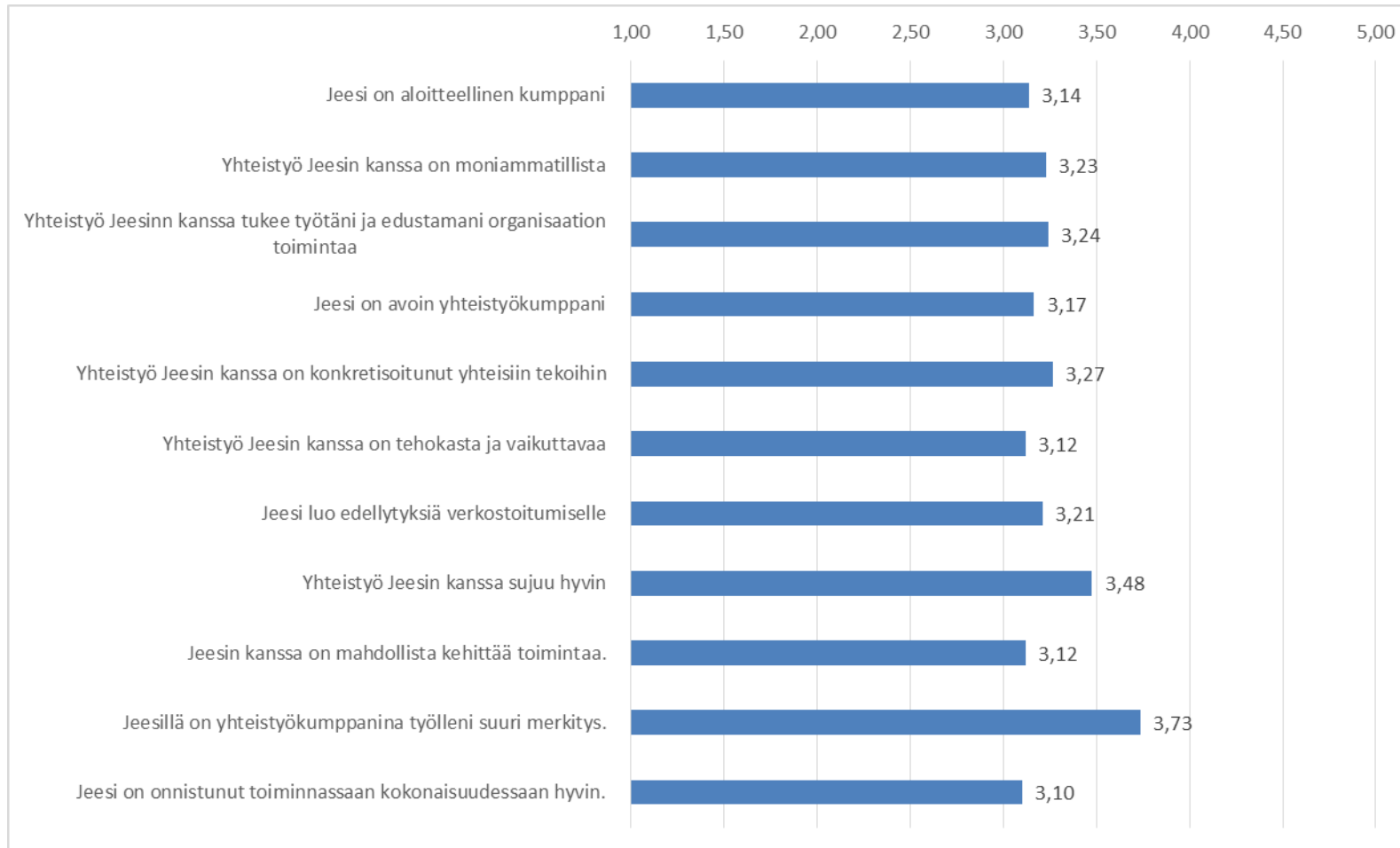
NPS-pisteet 21
