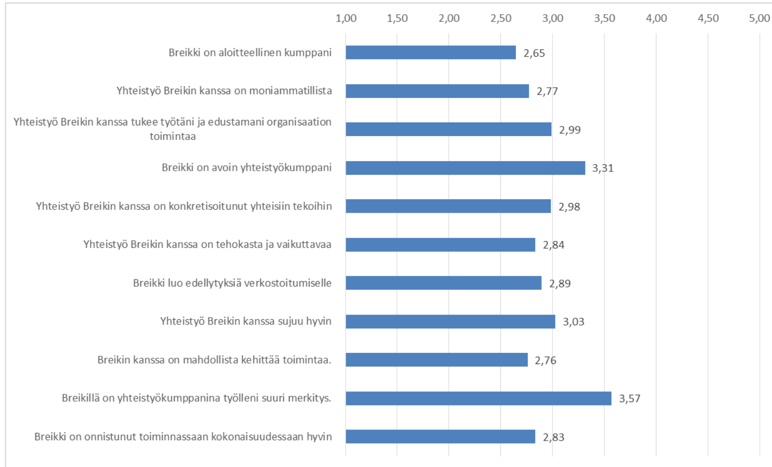
NPS-pisteet – 1
