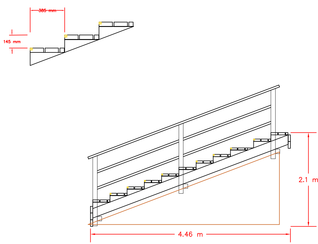
PORRAS 6 - 11 PORRASTA - NOUSU 145 mm - ETENEMÄ 385 mm
