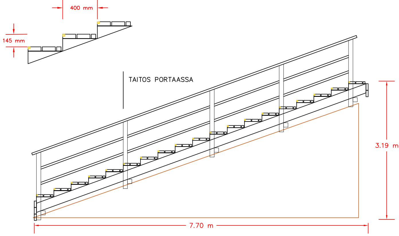
PORRAS 5 - 19 PORRASTA - NOUSU 145 mm - ETENEMÄ 400 mm
