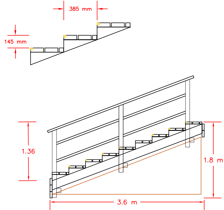
PORRAS 4 - 15 PORRASTA - NOUSU 145 mm - ETENEMÄ 385 mm
