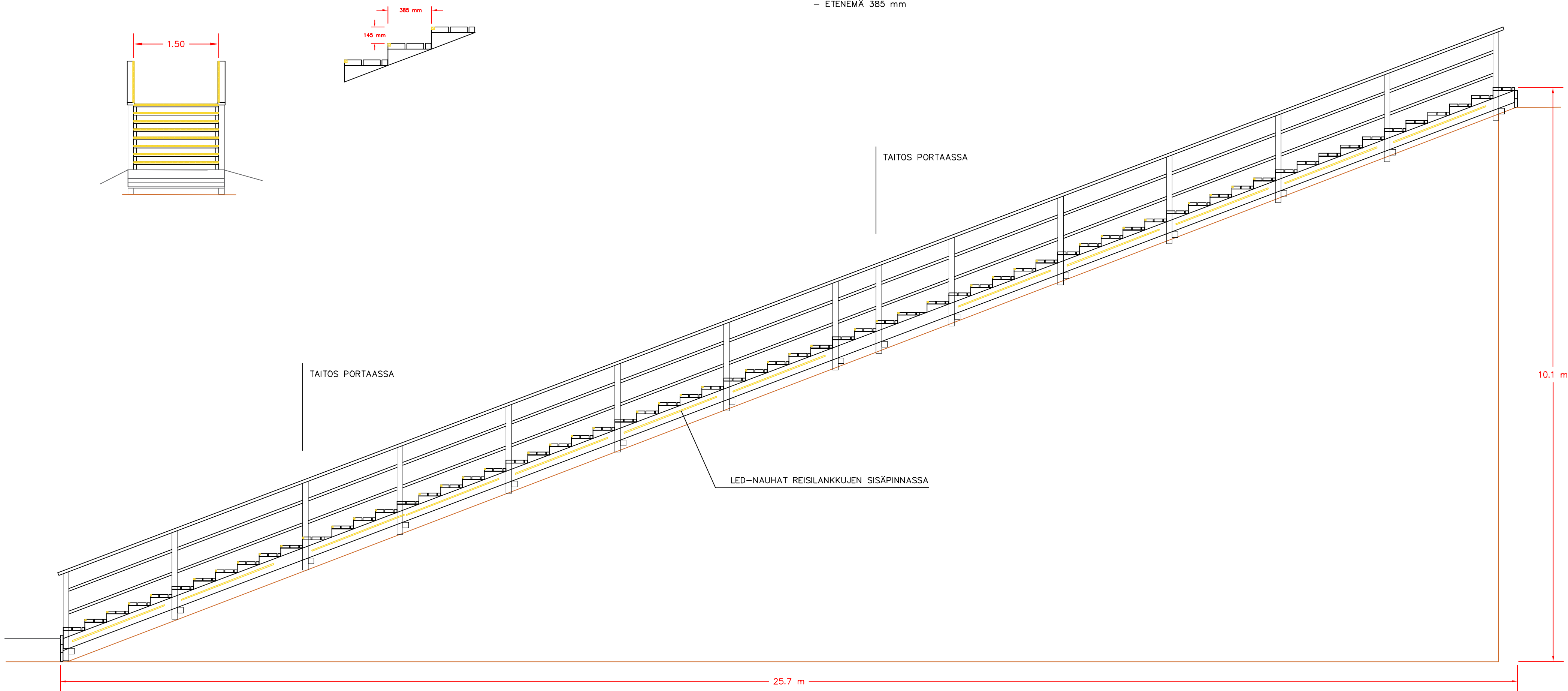
PORRAS 7 - 66 PORRASTA - NOUSU 145 mm - ETENEMÄ 385 mm
