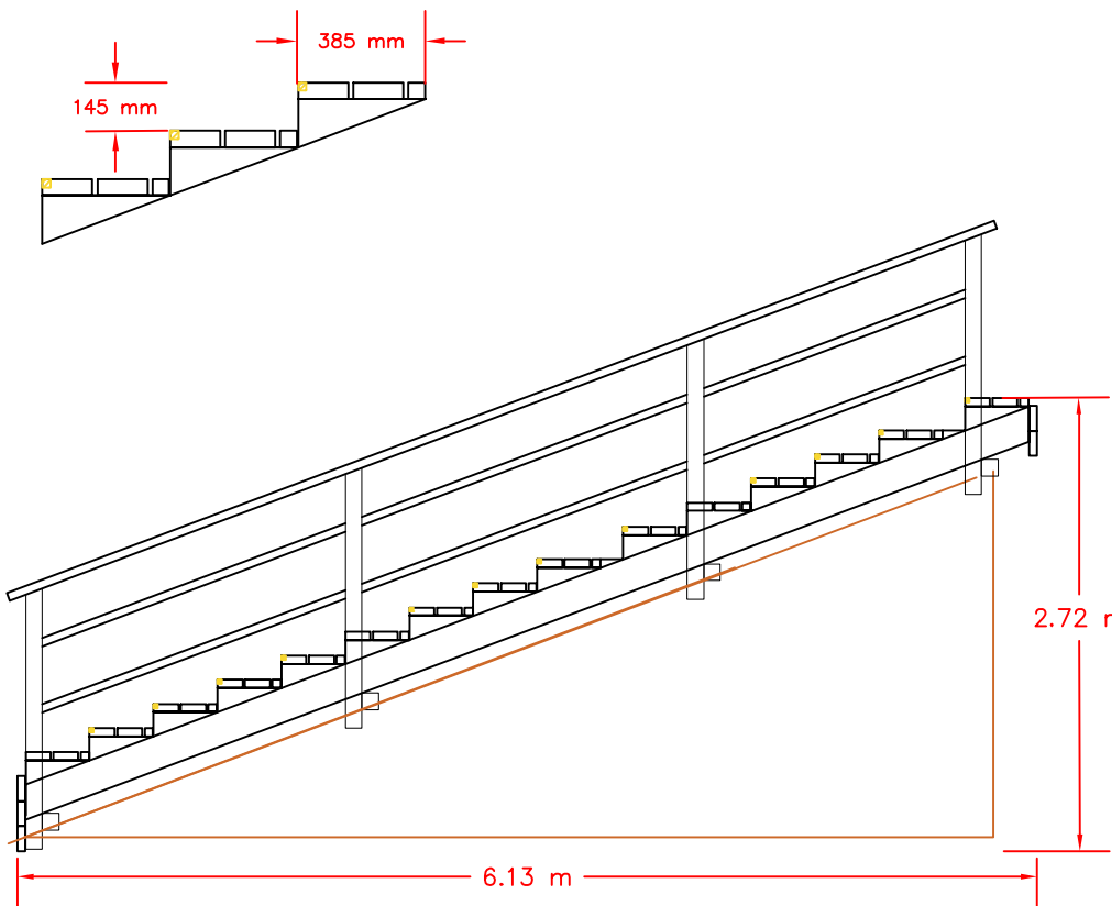
PORRAS 4 - 15 PORRASTA - NOUSU 145 mm - ETENEMÄ 385 mm
