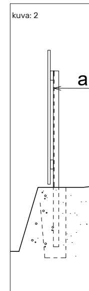
Puusäleaita yhdistettynä pulterimuuriin Pispalan valtatiellä
