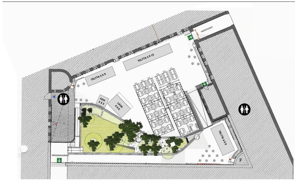
Kuva 1 Tapahtuma-alueen asemapiirros
