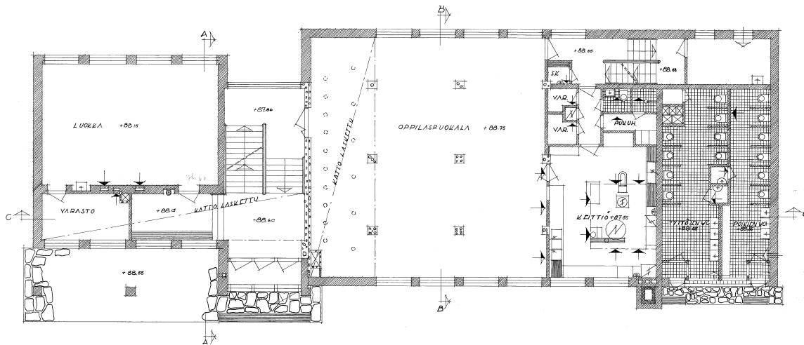
Pohjapiirros 1.kerros v. 1955
