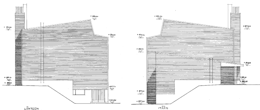
Päätyjulkisivut
