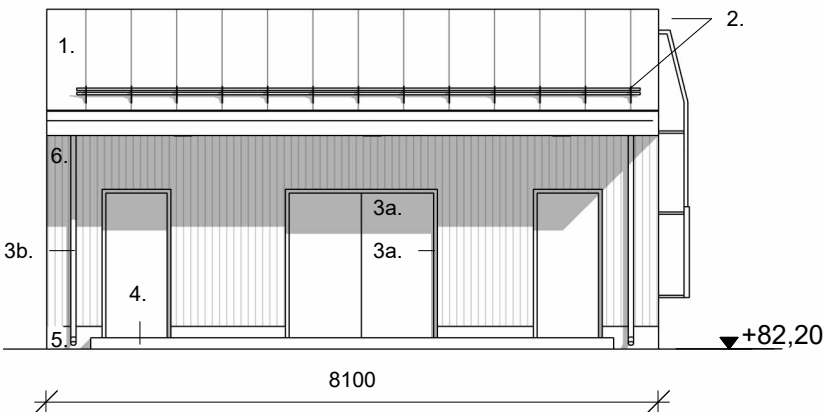
Itä 1 : 100
