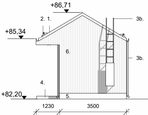
Pohjoinen 1 : 100
