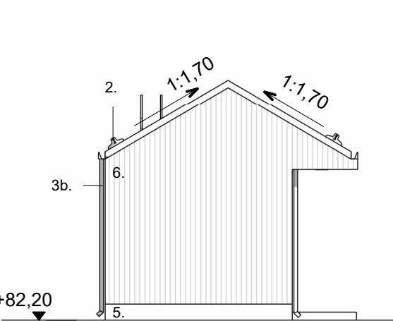
Pohjoinen 1 : 100
