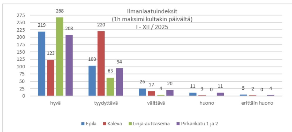
Kuva 8.1. Ilmanlaatu Tampereen eri asemilla (kunkin päivän 1 tunnin indeksien maksimi-arvon perusteella) mittausjakson aikana. Kaupunkitausta-asemalla Kalevassa otsonipitoisuus (jota muilla asemilla ei mitata) vähentää varsinkin kesäkaudella Kalevassa hyväksi luokitettujen päivien lukumäärää.
