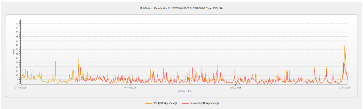
Kuva 4.3 Hiukkasten keuhkodepositoivan pinta-alan (LDSA) tuntikeskiarvoja ( \mu\text{m}^2/\text{cm}^3 ) Epilän ja Pirkankadun mittausasemilta.
