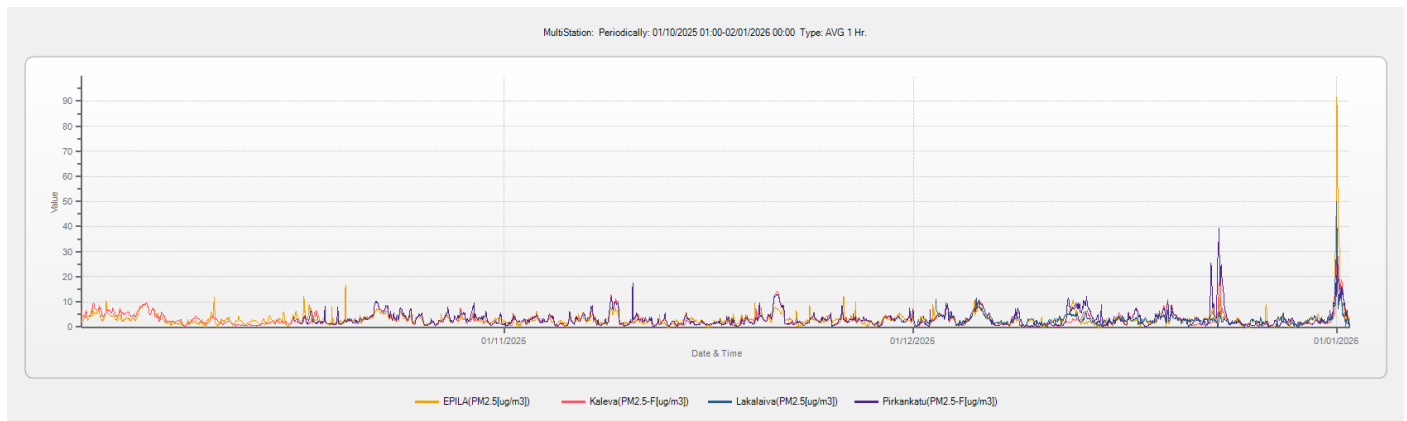
Kuva 3.2 Pienhiukkasten pitoisuuden tuntikeskiarvot mittausjakson aikana.
