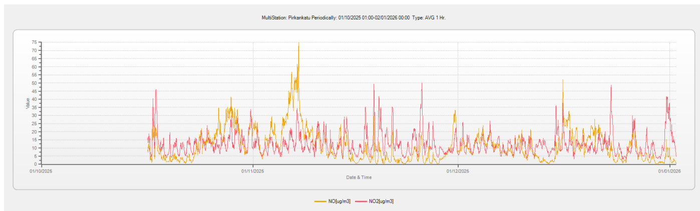
Kuva 5.3 Typen oksidien pitoisuuden tuntikeskiarvot Kalevassa, Linja-autoasemalla ja Pirkankadun asemilla mittausjakson aikana.
