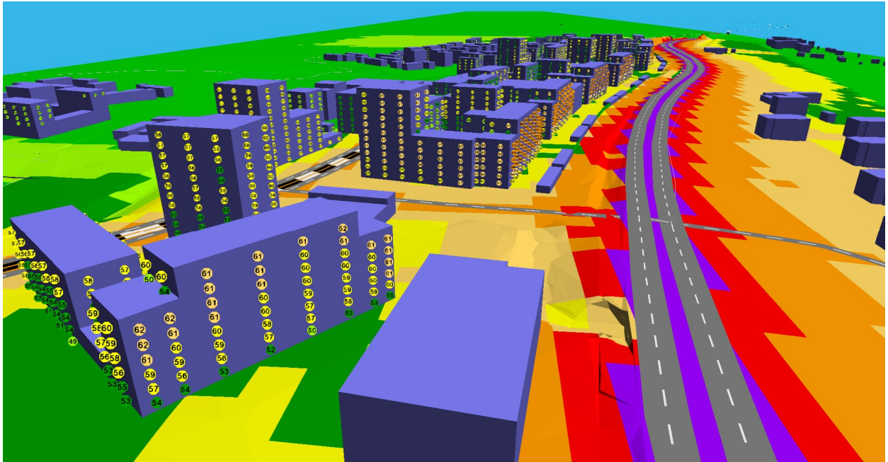
Kuva 1. Julkisivuihin kohdistuvat päiväaikaiset keskiäänitasot Teiskontien suunnasta.
