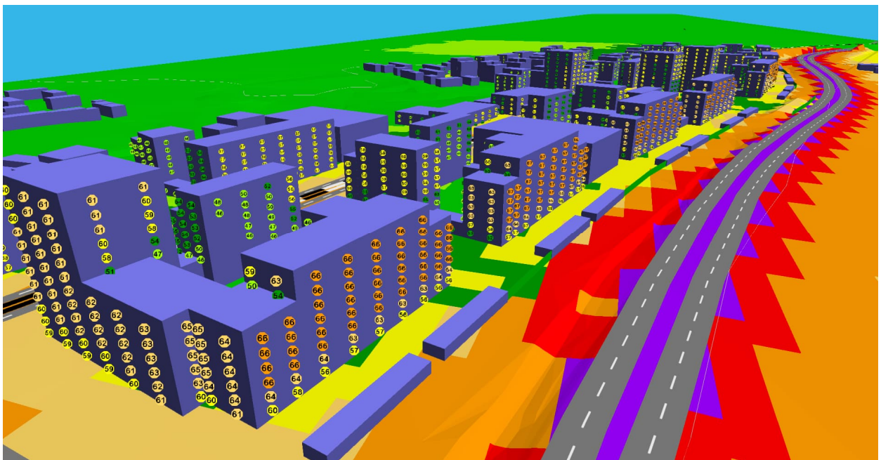
Kuva 2. Julkisivuihin kohdistuvat päiväaikaiset keskiäänitasot Teiskontien suunnasta.
