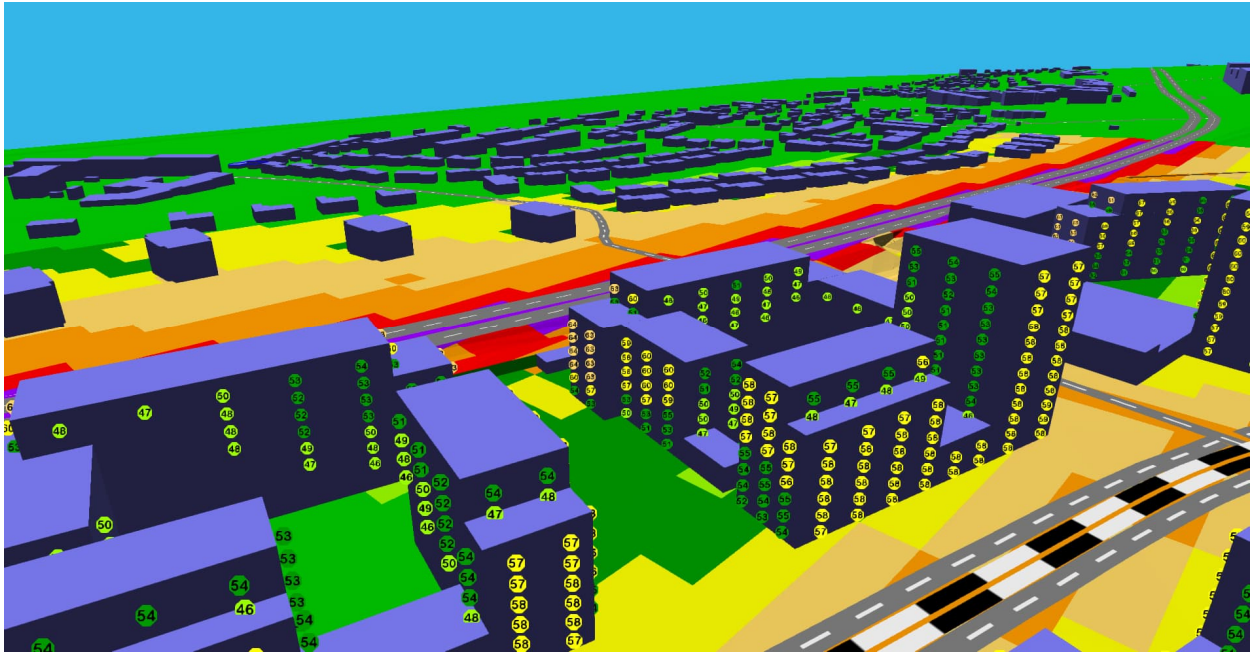
Kuva 7. Julkisivuihin kohdistuvat päiväaikaiset keskiäänitasot Kaupinlaakson Bulevardin suunnasta.
