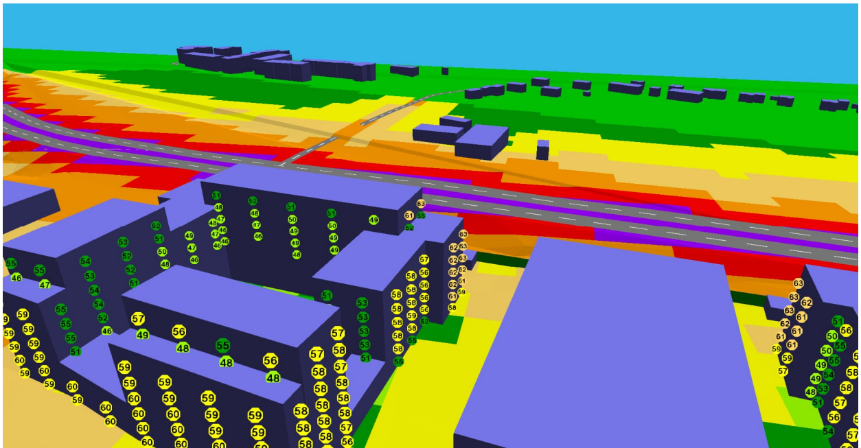
Kuva 10. Julkisivuihin kohdistuvat päiväaikaiset keskiäänitasot Kaupinlaakson Bulevardin suunnasta.
