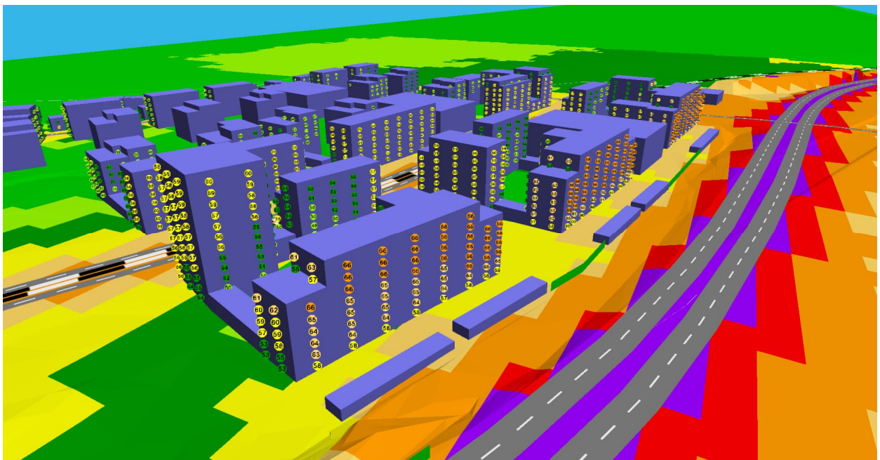
Kuva 4. Julkisivuihin kohdistuvat päiväaikaiset keskiäänitasot Teiskontien suunnasta
