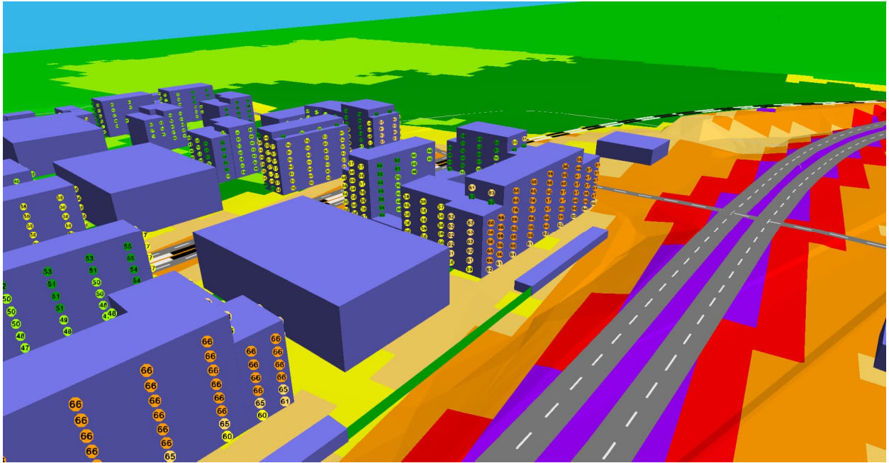
Kuva 5. Julkisivuihin kohdistuvat päiväaikaiset keskiäänitasot Teiskontien suunnasta.
