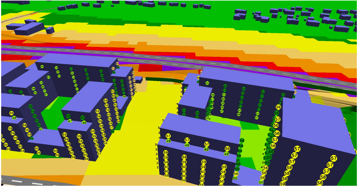
Kuva 9. Julkisivuihin kohdistuvat päiväaikaiset keskiäänitasot Kaupinlaakson Bulevardin suunnasta.
