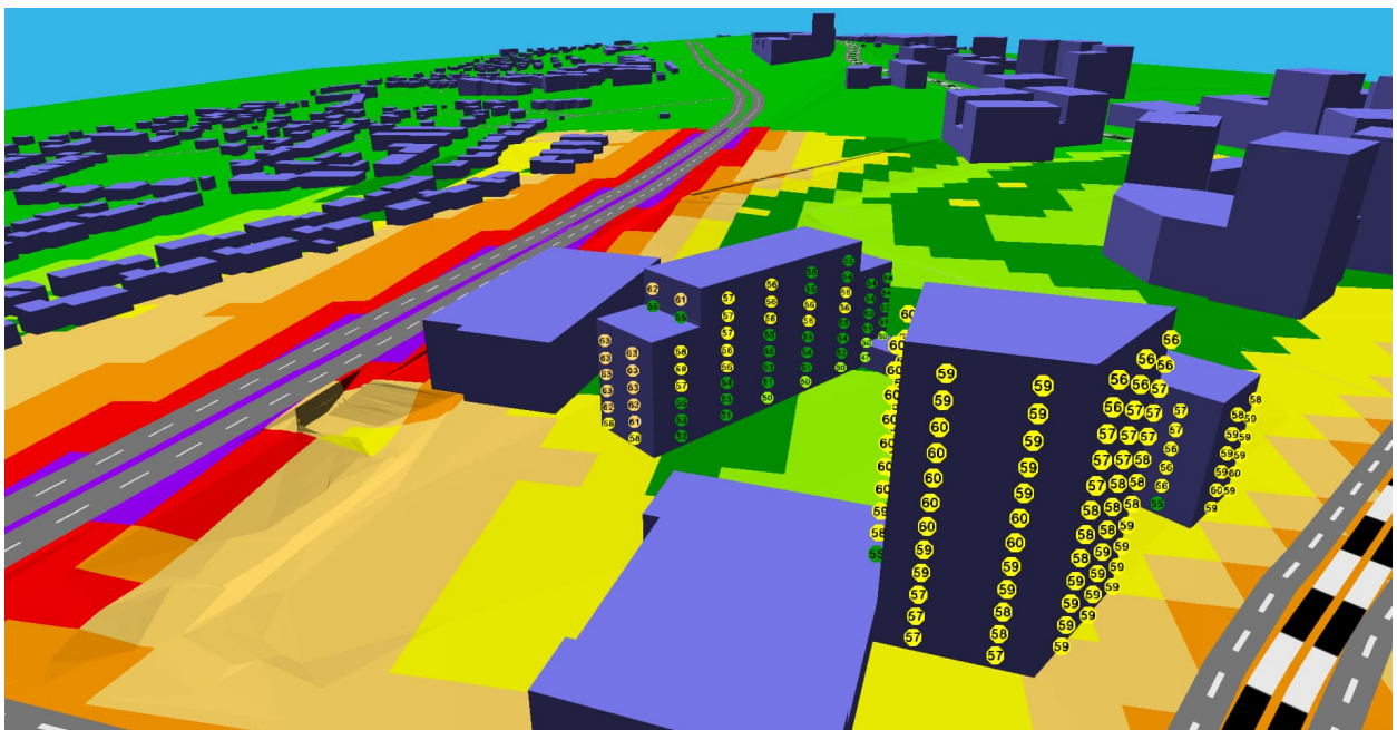
Kuva 6. Julkisivuihin kohdistuvat päiväaikaiset keskiäänitasot Kaupinlaakson Bulevardin suunnasta.
