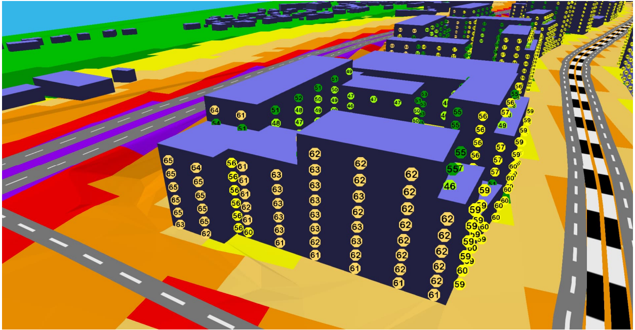
Kuva 11. Julkisivuihin kohdistuvat päiväaikaist keskiäänitasot Kaupinlaakson Bulevardin suunnasta.
