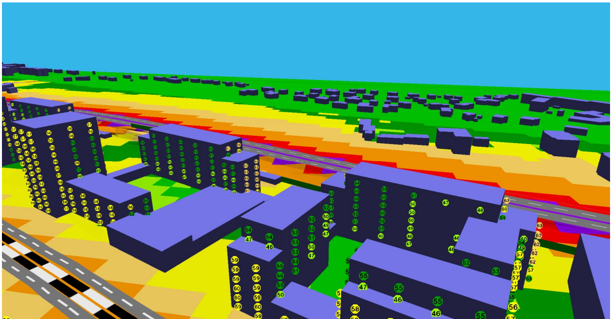
Kuva 8. Julkisivuihin kohdistuvat päiväaikaiset keskiäänitasot Kaupinlaakson Bulevardin suunnasta.
