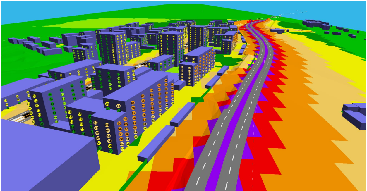
Kuva 3. Julkisivuihin kohdistuvat päiväaikaiset keskiäänitasot Teiskontien suunnasta
