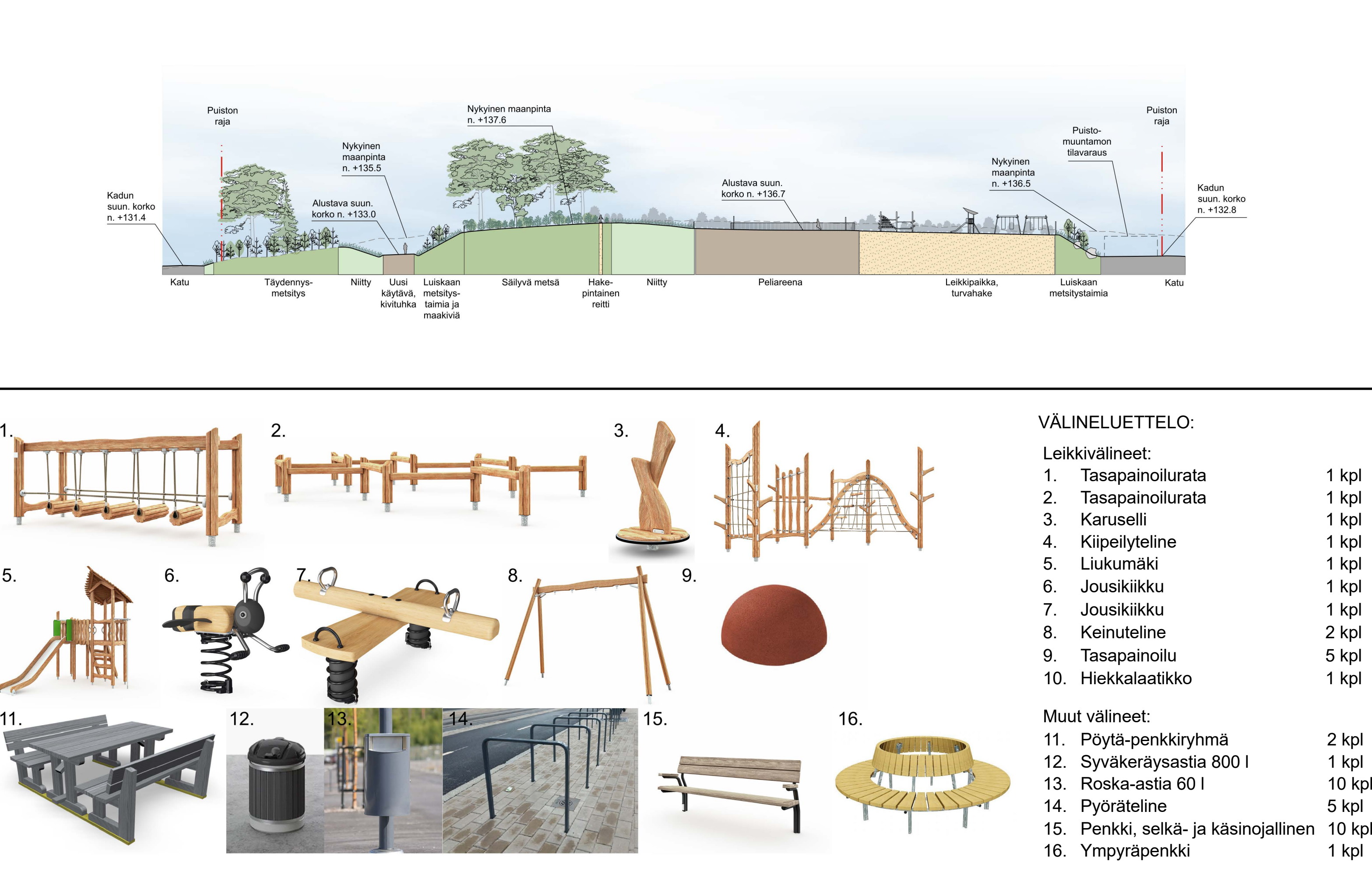
LEIKKAUS A-A 1:500
