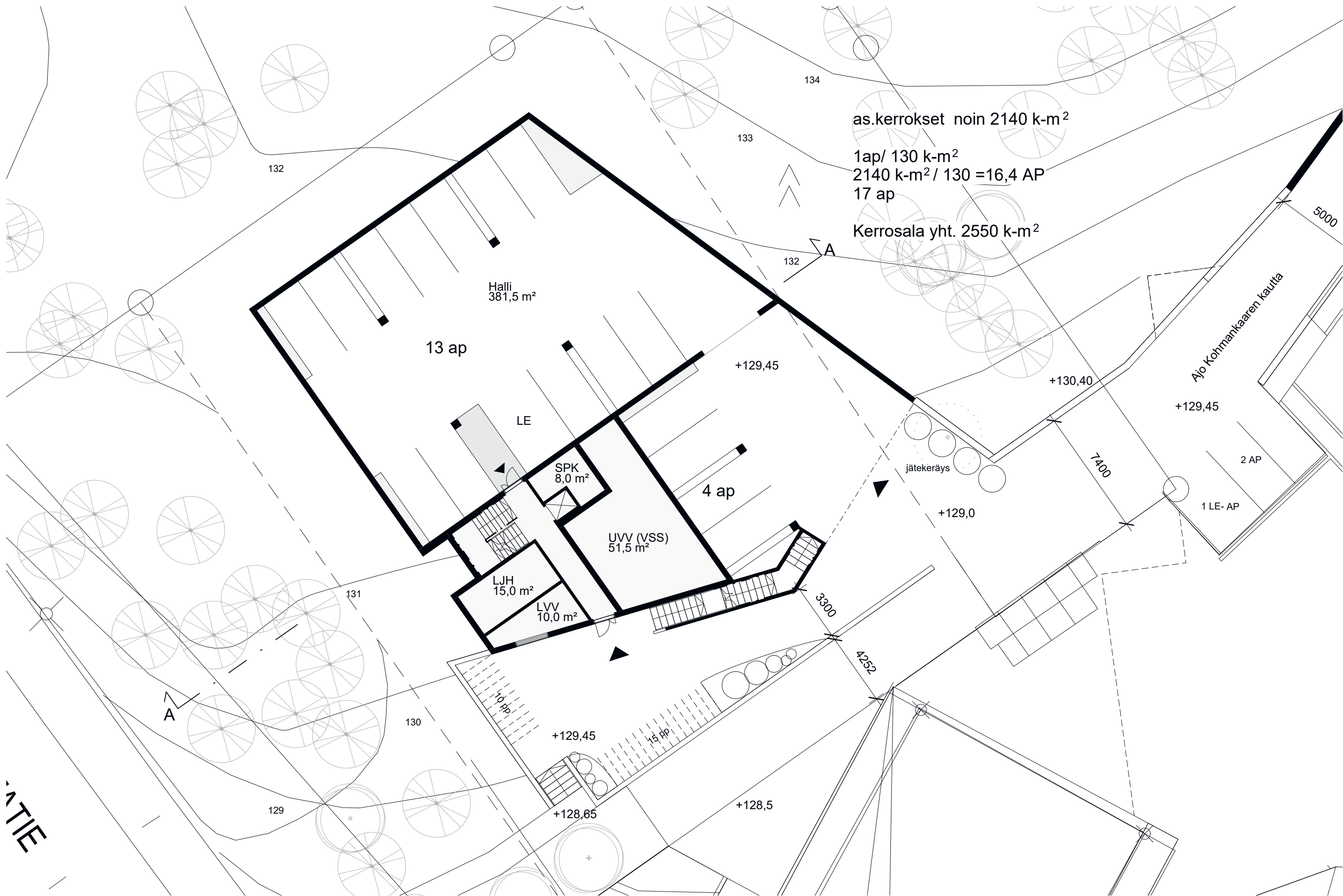
0. krs pohjapiirros (maantaso) 1:200
