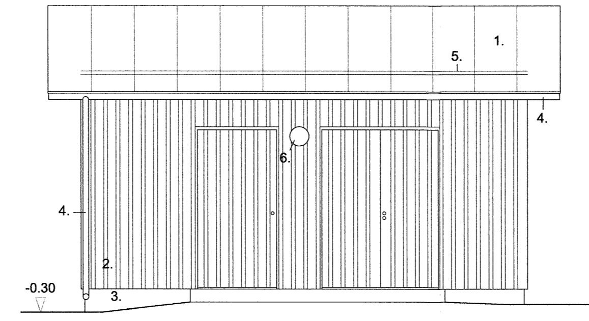
JULKISIVU ITÄÄN 1:50
