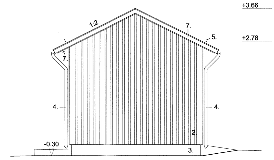
PÄÄDYT 1:50
