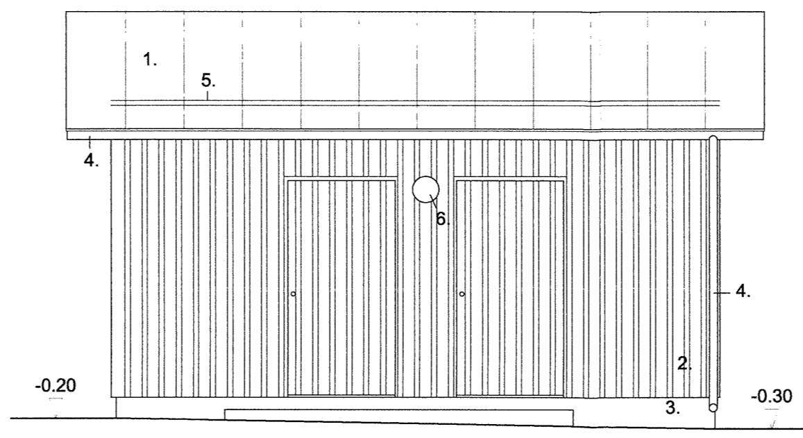
JULKISIVU LÄNTEEN 1:50
