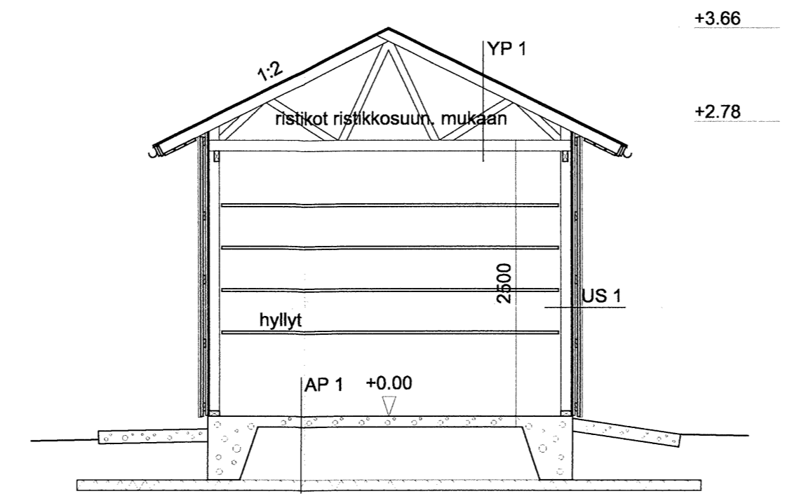
LEIKKAUS A-A 1:50
