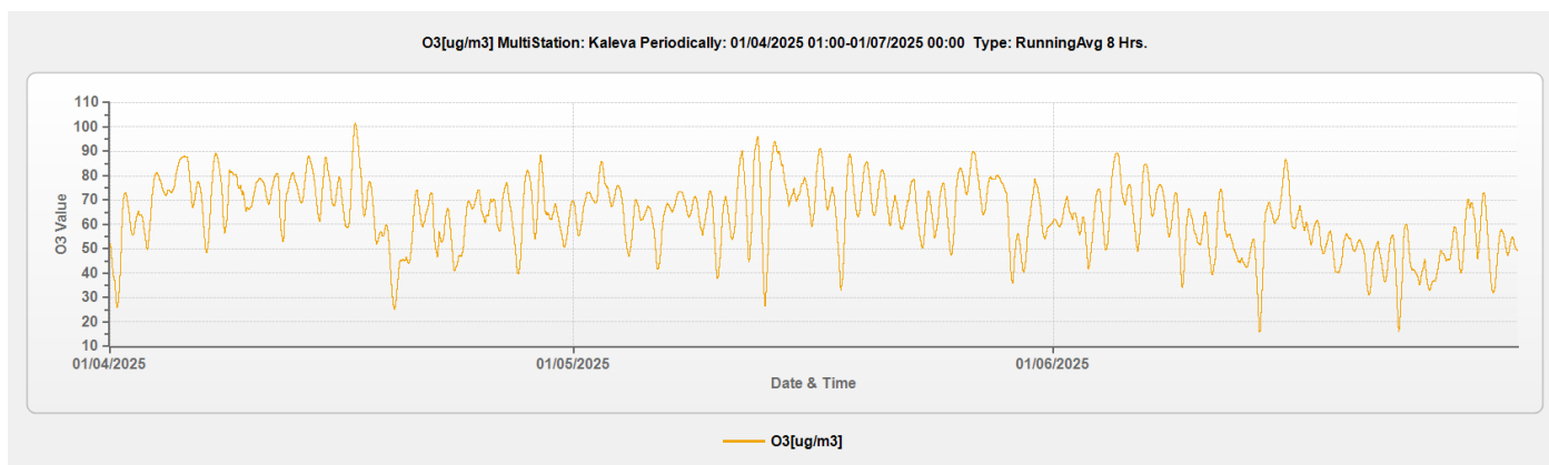
Kuva 6.1 Otsonipitoisuuden (liukuvat) 8h -keskiarvot Kalevan mittausasemalla.
