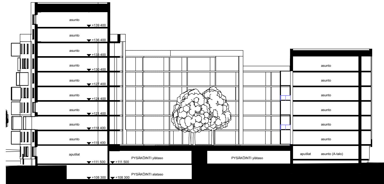
Periaateleikkaus
