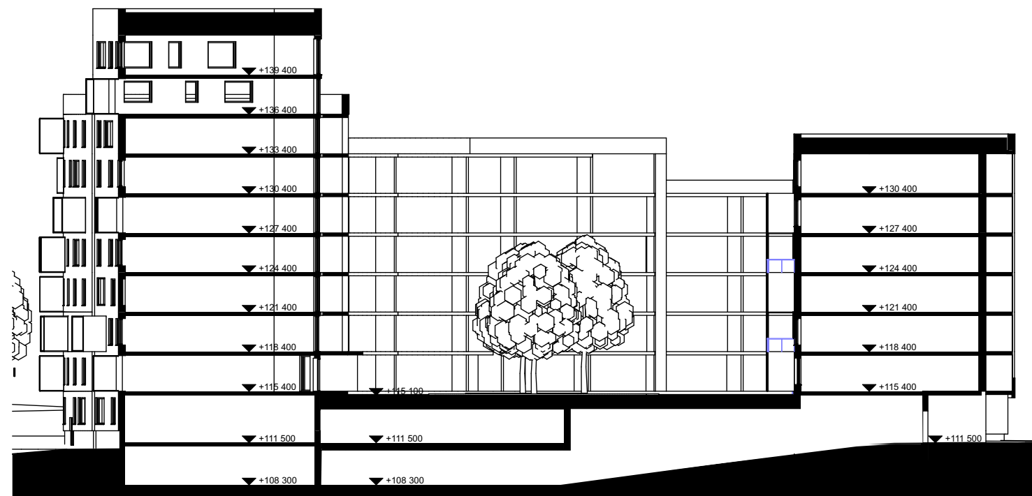
Periaateleikkaus alatasen sisäänajoluiskan kohdalta
