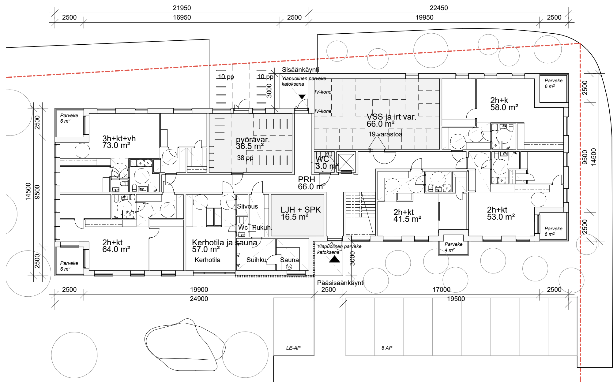
Pohjapiirros 1. krs.
