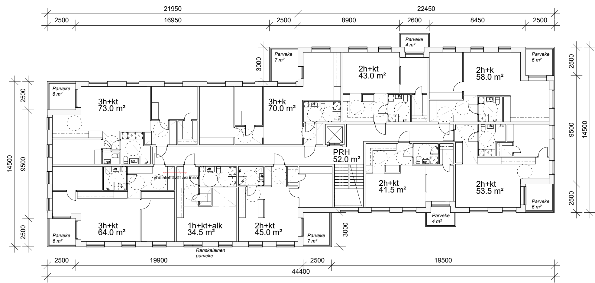
Pohjapiirros 2-5. krs.
