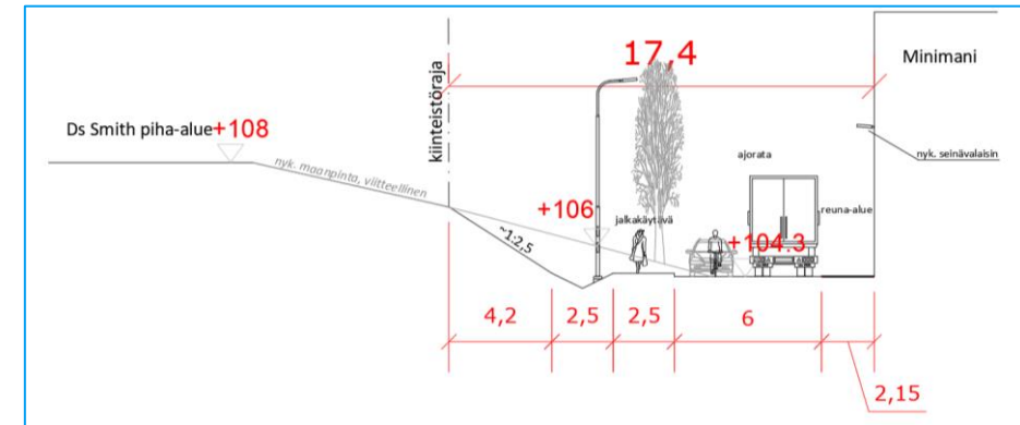
Leikkaus A-A, Minimanin koillispuolelta, vaihtoehdot VE1A, VE1B ja VE2.
