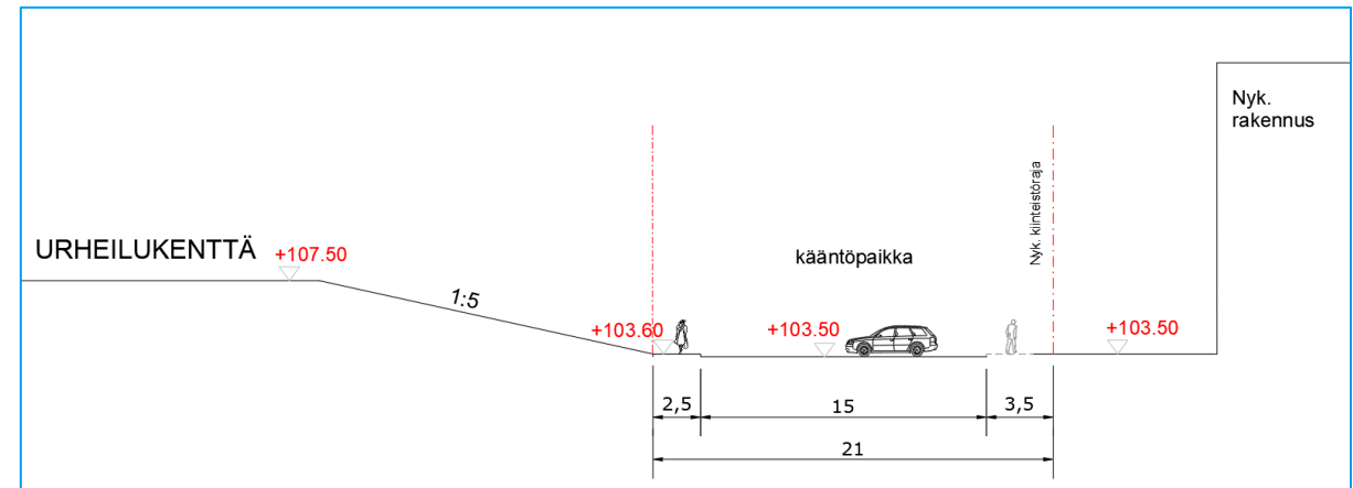
Leikkaus E-E
