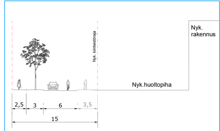
Leikkaus B-B
