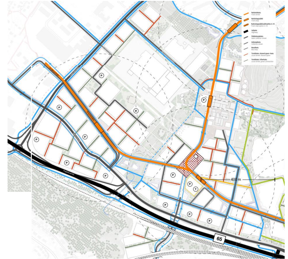
Hiedanrannan yleissuunnitelman kortteli- ja katuverkkorakenne.
