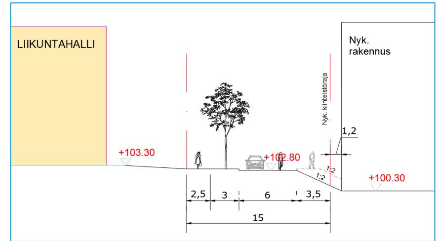
Leikkaus C-C
