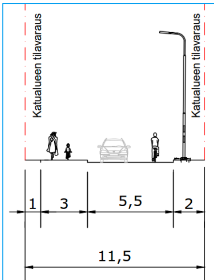
Leikkaus H-H
