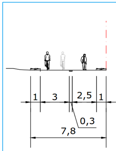
Leikkaus I-I
