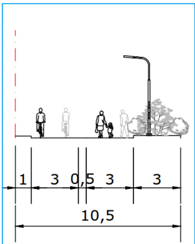
Leikkaus G-G
