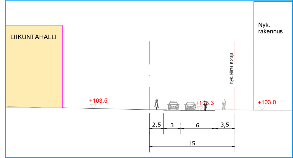
Leikkaus D-D
