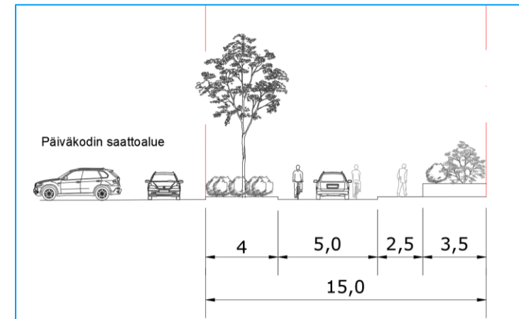
Leikkaus F-F
