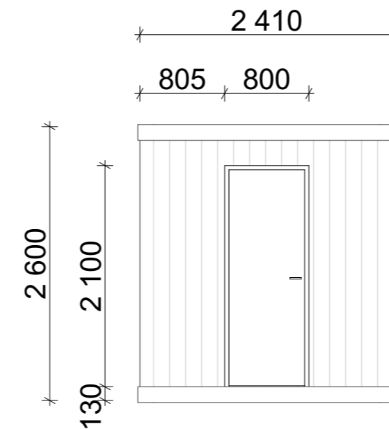
1:50 Julkisivu D
