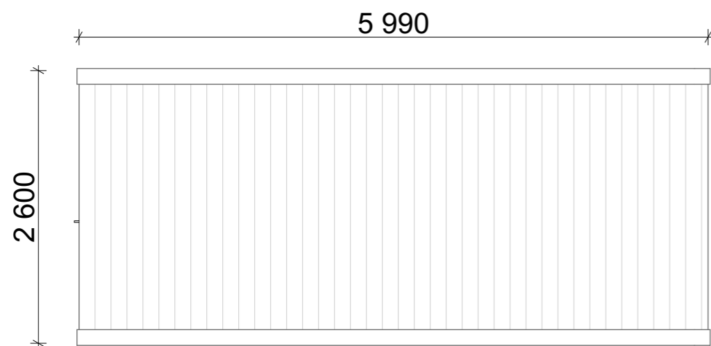
1:50 Julkisivu C
