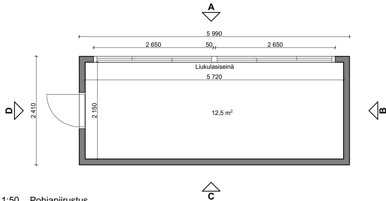
1:50 Pohjapiirustus
