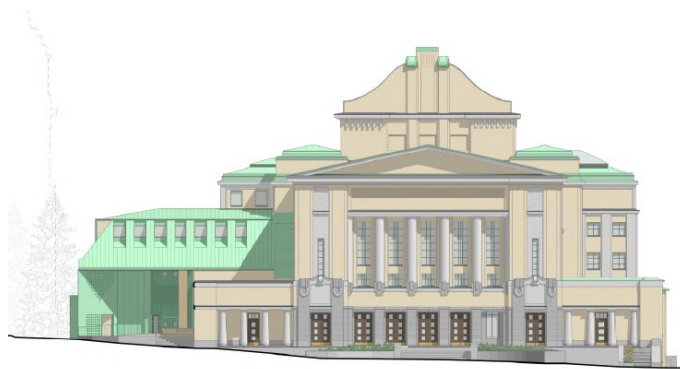
Kuva 31 Teatterin julkisivukuvassa länteen Keskustorille päin on kuvattu aloitusvaiheessa nähtävillä ollut laajennuksen viitesuunnitelma. Laajennus sijoittuu teatterin pohjoispuolelle ja on kuvassa vasemmalla. Hissiyhteys on sijoitettu teatterirakennuksen sisälle porrashuoneeseen.
