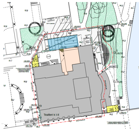
Kuva 29 Teatterin laajennus ja pystynousujen tarkastelu. Piirroksessa on esitetty harmaalla nykyinen teatterirakennus ja vaaleanruskealla teatterin uusi laajennus. Sinisellä värillä on kuvattu maanalaisen kaavan 8437 aineistoissa esitetty mahdollinen nousujen sijoitusalue. Lisäksi keltaisella on esitetty teatterin viitesuunnitelman yhteydessä tutkitut vaihtoehdot pystynousujen sijainnit.
