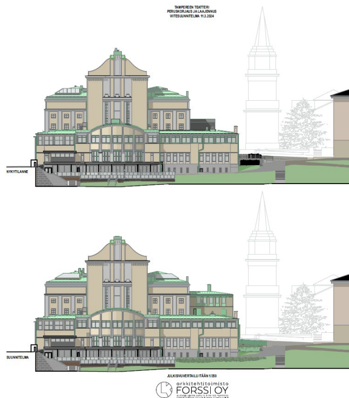
Kuva 26 Julkisivu itään Tammerkoskelle päin, yllä nykytila ja alla viitesuunnitelman mukainen ratkaisu. Oikealla on kuvattu Kulttuuritalo Laikku ja taustalla vaalealla viivalla kellotapuli. 1939-luvun laajennus on teatterin päämassasta oikealla. Teatterin uusi laajennus erottuu koski- ja puistomaisemassa, mutta jää osittain olemassa olevan puuston taakse kauempaa tarkasteltuna.
