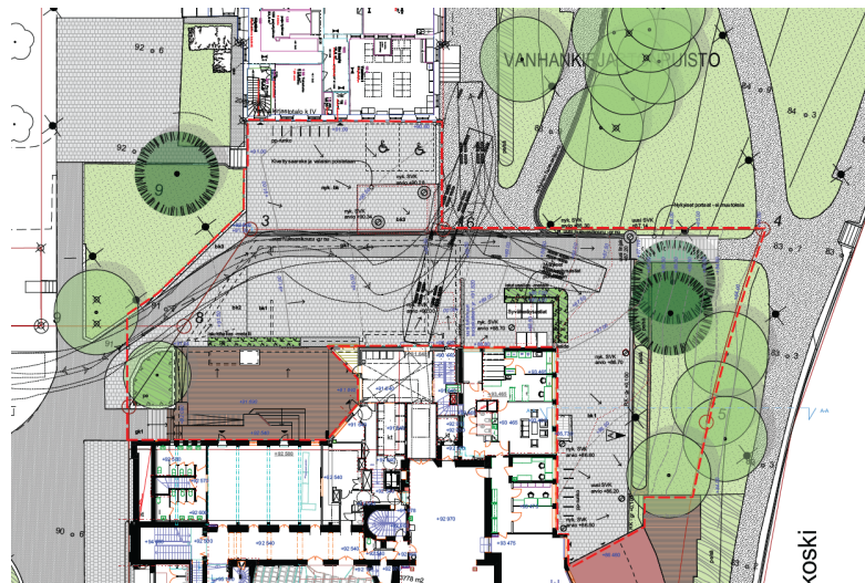
Kuva 34 Ote pihasuunnitelmasta, Sitowise 11.3.2024. Pihasuunnitelmassa on esitetty teatterin piha-alueen järjestelyt sekä ajoneuvojen ajouratarkastelu ja tilavaraukset.
