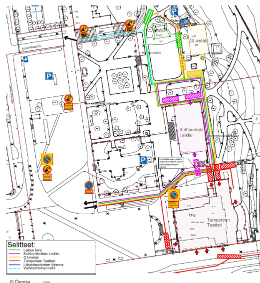
Kuva 35 Kaavio Tampereen teatterin ja puistoalueen huoltoliikenteen tavoitetilasta. Destia, 2023. Huoltoliikenteen reitit on esitetty eri väreillä. Teatterin ja Laikun kulttuuritalon tonttien kautta on huoltoyhteyden tarve teatterin ja Laikun kulttuuritalon lisäksi G Livelabilla ja Laikunlavalla.
