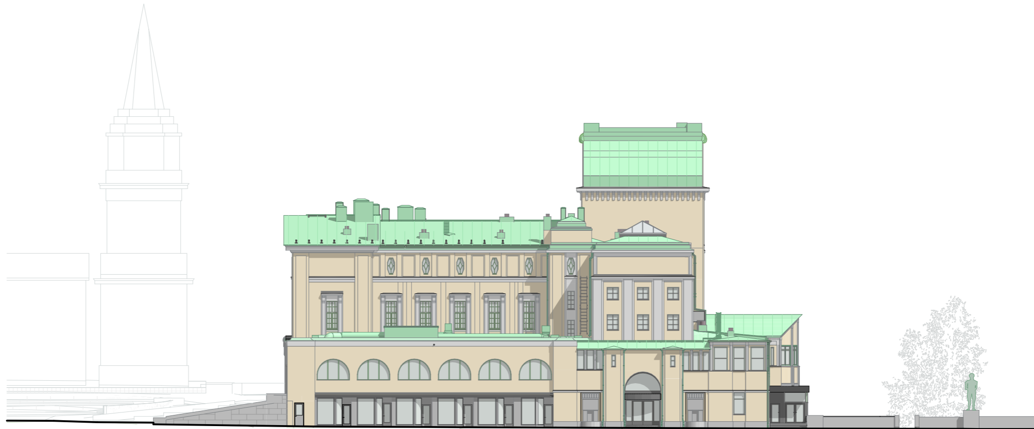
JULKISIVUVERTAILU ETELÄÄN 1/350
