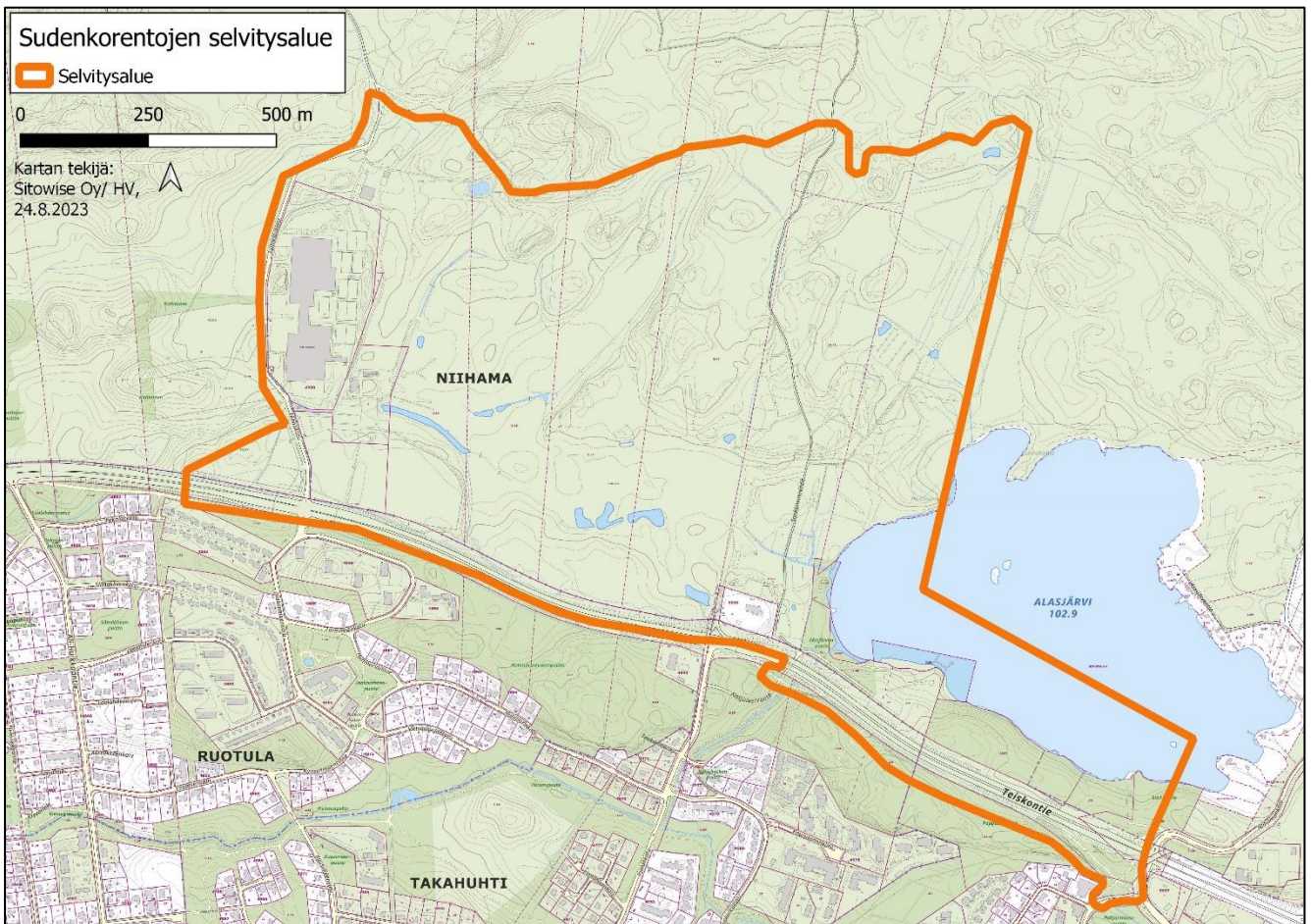
Kuva 1. Selvitysalueen rajaus.
