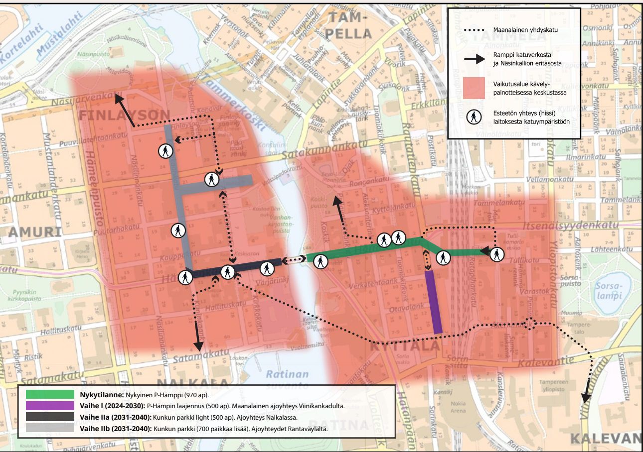
Kuva 5.2 Tampereen keskustan maanalaisen periaatteena on autoilijalle autokehän helppo saavutettavuus ja siitä vaivaton siirtyminen pysäköintilaitoksiin. Pysäköintilaitoksesta on esteetön ja turvallinen siirtyminen katuymppäristöön. Autoa voi esteettä siirtää maanalaisessa pysäköintiverkossa itäosasta länsiosaan.
