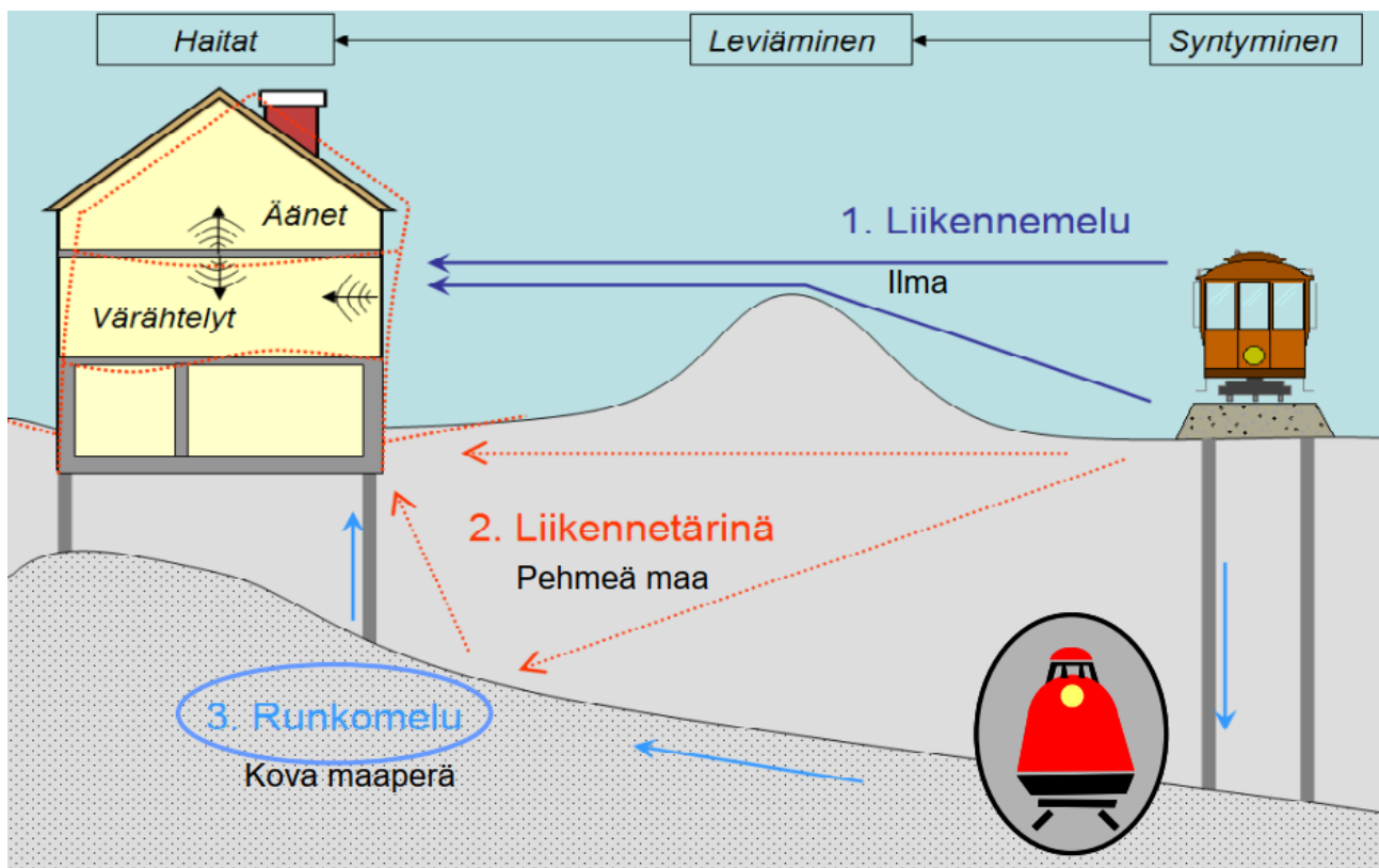
Kuva 3. Tärinän ja runkomelun syntyminen, leviäminen ja vaikutukset ympäristöön (Tajja & Saarinen 2009).
