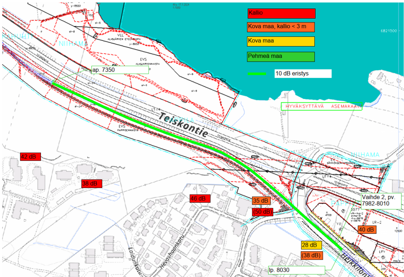
Kuva 11 Laskennalliset runkomelutasot ilman runkomelueristystä ja esitetty runkomeluvaimennus kiskonaluslevyjen lisäksi paaluvälillä 7350 – 8000. Sulkeissa olevat arvot mahdollisia, mikäli rata ja/tai rakennus on kallionvarainen. Tausta-aineistona Tampereen virastokartta sekä valmisteluvaiheen asemakaavat 8933 ja 8876.
