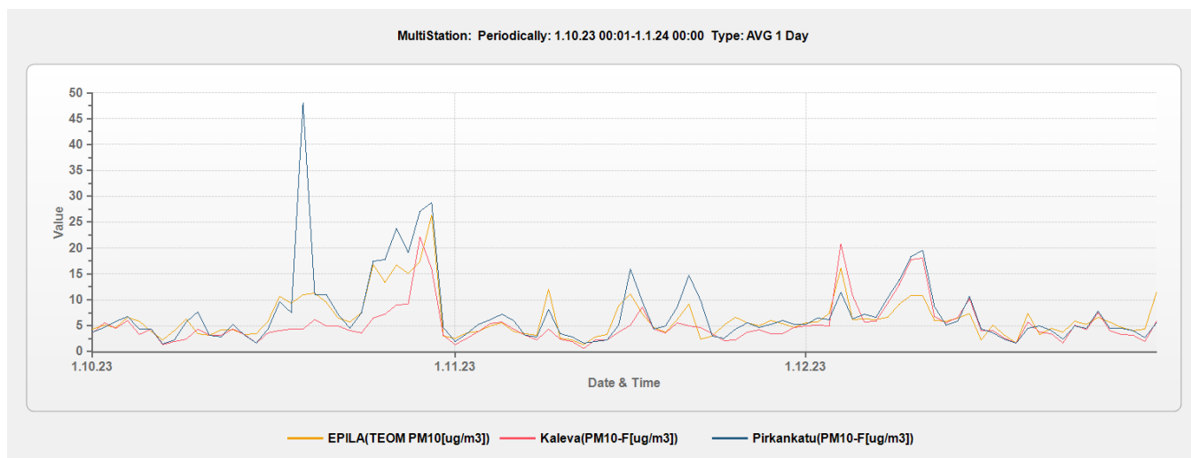
Kuva 2.2 Hengitettävien hiukkasten pitoisuuden vuorokausikeskiarvoja mittausjakson aikana Epilässä, Kalevassa ja Pirkankadulla.
