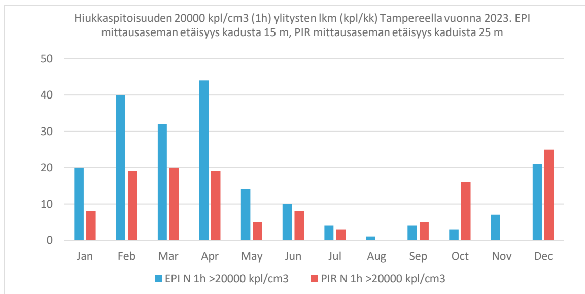
Kuva 4.6 Jatkuvatoimisissa mittauksissa havaittujen hiukkasten lkm-pitoisuuksien tuntikeskiarvon 20000 kpl/cm 3 ylitysten lukumäärä (kpl/kk) vuonna 2023 Epilän (yht. 200 kpl/a) ja Pirkankadun (yht. 128 kpl/a) mittausasemilla. WHO:n kannanoton (taulukko 4.1) mukaan hiukkasten lukumääräpitoisuus on korkea, kun pitoisuuden 1h keskiarvo on yli 20000 kpl/cm 3 . Mittaukset on tehty asemien seinustoille sijoitetuilla AQ Urban sensoreilla.
