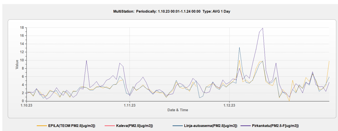
Kuva 3.1 Pienhiukkasten pitoisuuden vuorokausikeskiarvot mittausjakson aikana Epilässä ja Linja-autoasemalla (Teom) ja Kalevassa ja Pirkankadulla (Fidas).
