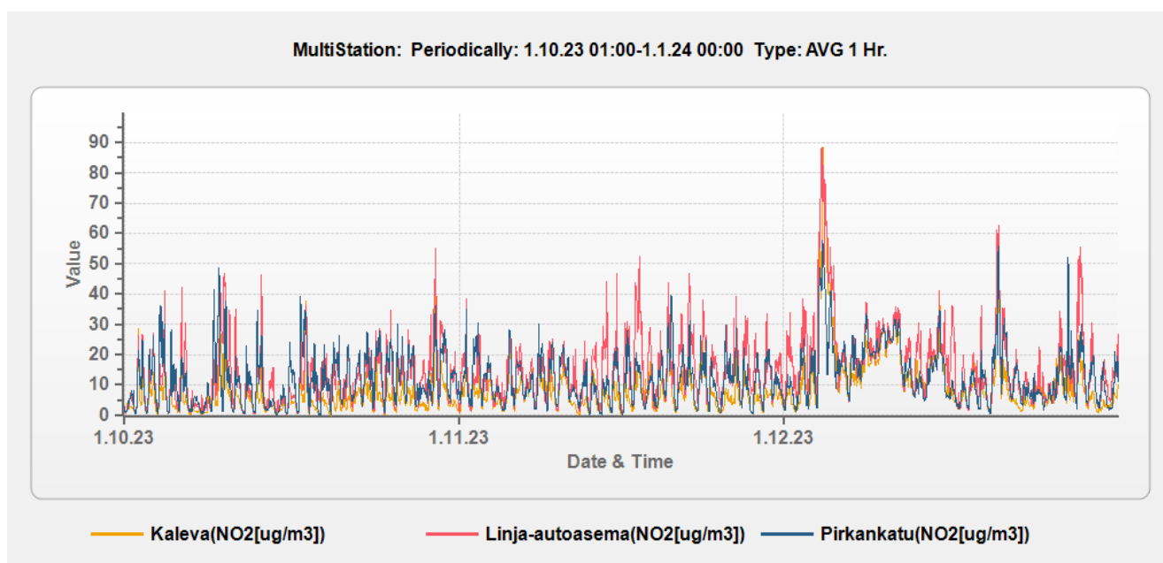
Kuva 5.2 Typpidioksidin pitoisuuden tuntikeskiarvot Kalevassa, Linja-autoasemalla ja Pirkankadulla mittausjakson aikana.
