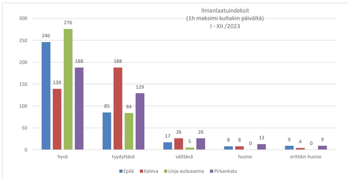
Kuva 8.1. Yhteenveto ilmanlaadusta Tampereen eri asemilla (kunkin päivän 1 tunnin maksimiarvon perusteella) kuluneen vuoden aikana. Kaupunkitausta-asemalla Kalevassa otsonipitoisuus (jota muilla asemilla ei mitata) vähentää varsinkin kesäkaudella Kalevassa hyväksi luokitettujen päivien lukumäärää.
