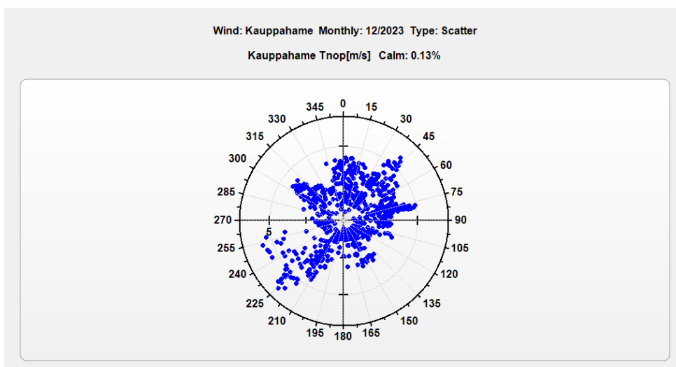
Kuva 7.2 Tuulen nopeus suunnittain 1h keskiarvoina Kauppa-Hämeen sääasemalta.
