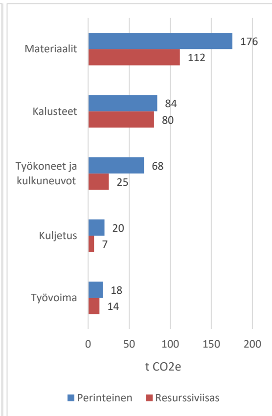
Kuva 31. a) Perinteisen ja resurssiviisaan kadun saneerauksen aiheuttama luontojalanjälki (nPDF) ja b) perinteisen ja resurssiviisaan kadun saneerauksen aiheuttama hiilijalanjälki (t CO 2 e).
