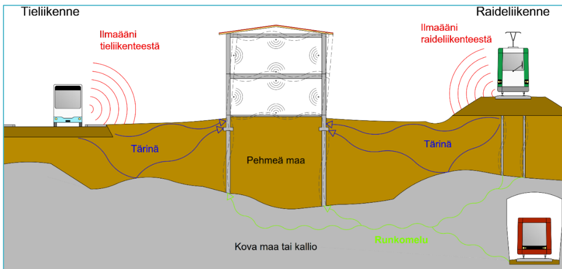
Kuva 2.1. Periaatekuva raideliikenteen aiheuttaman värinän ja runkomelun etenemisestä eri maalajeissa.
