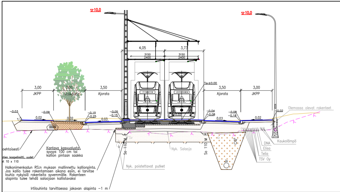
Kuva 4.2. Raitiotien tyyppipoikkileikkaus, Halkoniemenkatu PLV 100-137, Ratapaalu 6606-6643 (saatu ÅFRY:lta 29.8.2023).
