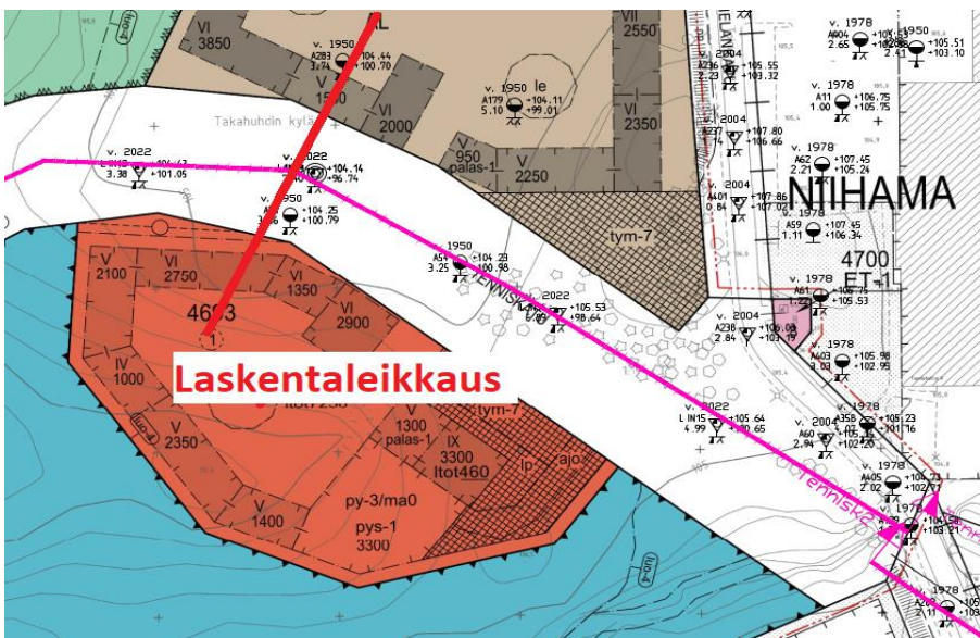
Kuva 4. Tärinälaskennan leikkauksen Medi-Park IV sijainti (punainen viiva).
