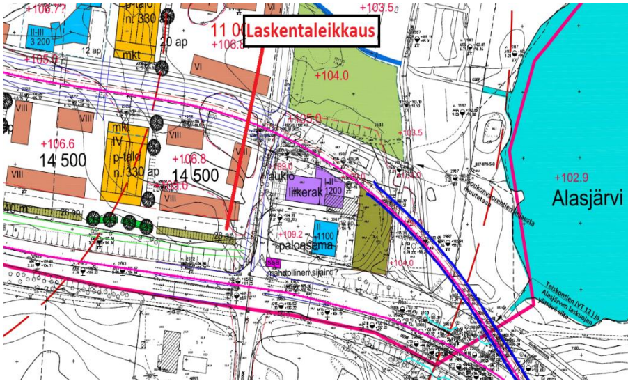
Kuva 3. Tärinälaskennan leikkauksen Alasjärvi läntinen sijainti (punainen viiva).
