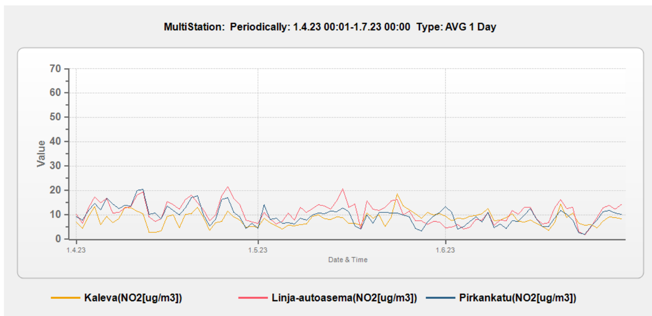
Kuva 5.1a Typpidioksidin pitoisuuden vuorokausikeskiarvot eri mittausasemilla mittausjakson aikana.
