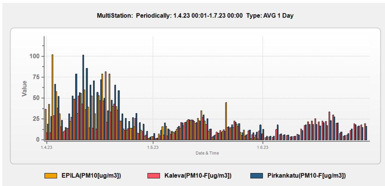
Kuva 2.1 Hengitettävien hiukkasten pitoisuuden vuorokausikeskiarvot mittausjakson aikana Epilässä, Kalevassa ja Pirkankadulla. Epilän Grimm-laite oli huollossa 1.6. alkaen.
