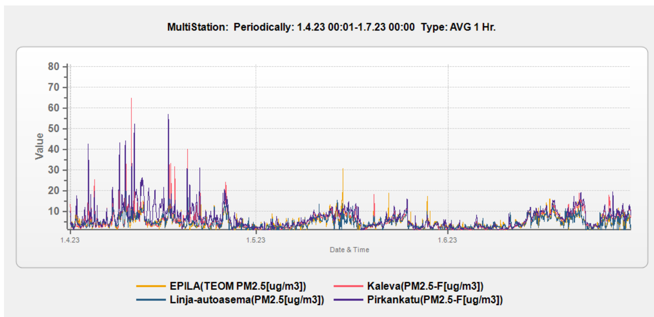
Kuva 3.2 Pienhiukkasten pitoisuuden tuntikausikeskiarvot mittausjakson aikana Epilässä (Teom), Kalevassa, Linja-autoasemalla (Teom) ja Pirkankadulla. Epilän Grimm-laitte oli huollossa 1.6. alkaen.
