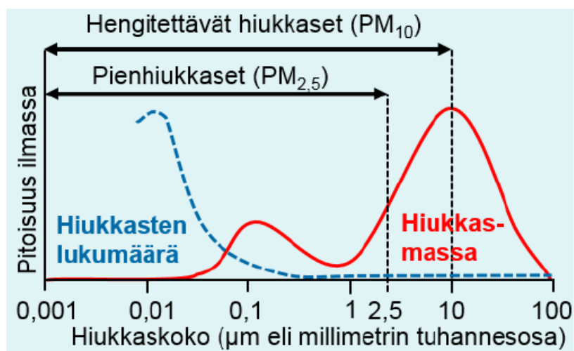
Kuva 2.1a Hiukkaskoko vs. lukumäärä – ja massapitoisuus (Julkunen 2016). Ultrapientien hiukkasten halkaisija alle 0,1 \mu\text{m} .
