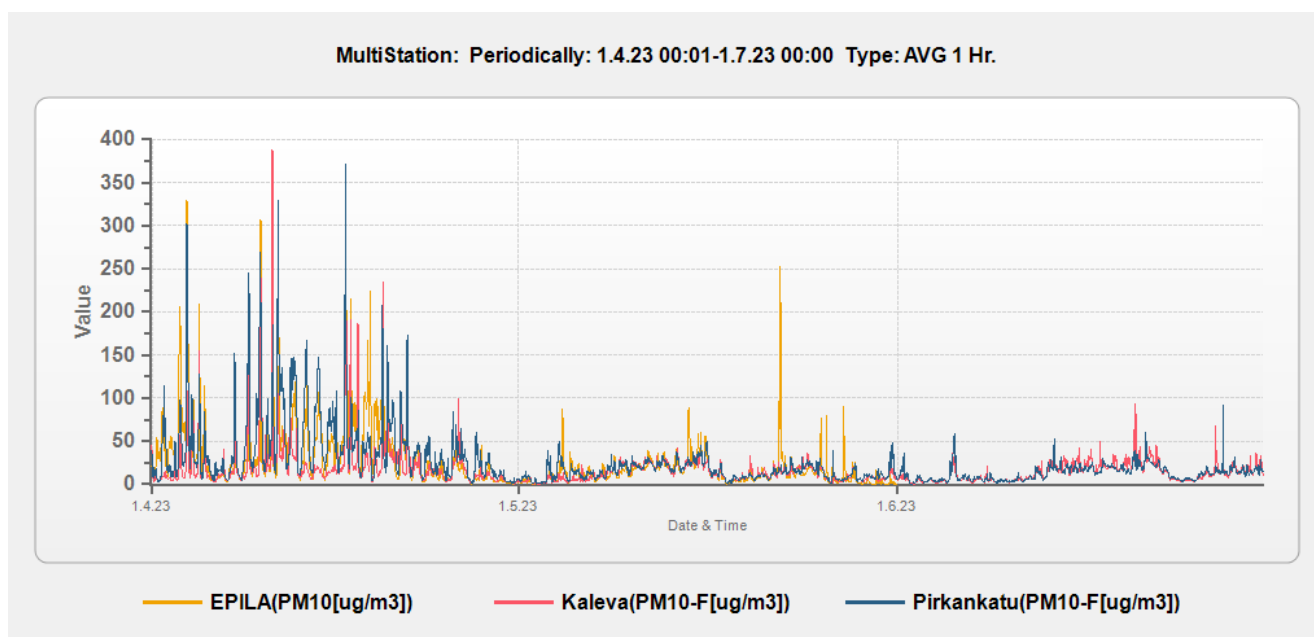
Kuva 2.3 Hengitettävien hiukkasten pitoisuuden tuntikeskiarvot Epilässä, Kalevassa ja Pirkankadulla mittausjakson aikana. Epilän Grimm-laite oli huollossa 1.6. alkaen.
