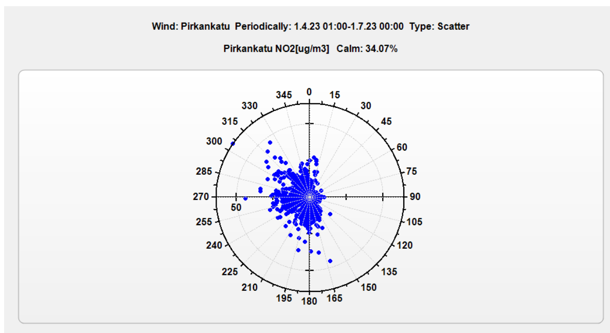
Kuva 5.1b Typpidioksidin pitoisuuden tuntikeskiarvot Pirkankadulla tuulensuunnittain mittausjakson aikana.
