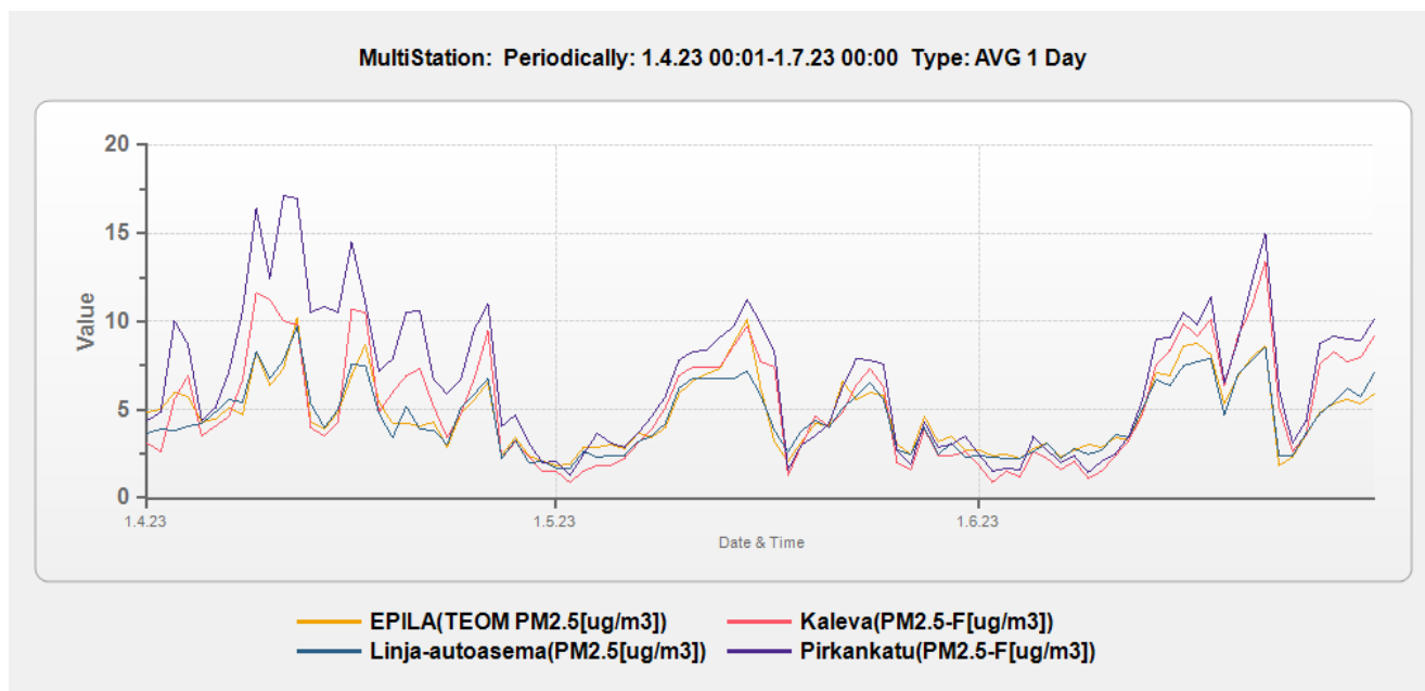
Kuva 3.1 Pienhiukkasten pitoisuuden vuorokausikeskiarvot mittausjakson aikana Epilässä (Teom), Kalevassa, Linja-autoasemalla (Teom) ja Pirkankadulla. Epilän Grimm-laitte oli huollossa 1.6. alkaen.
