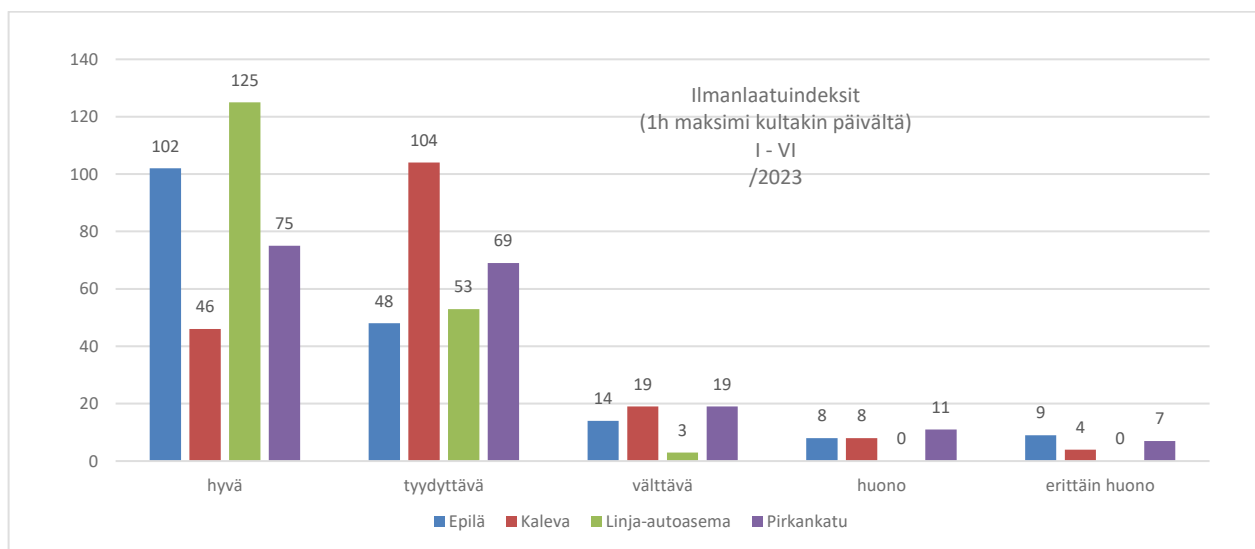
Kuva 8.1. Yhteenveto ilmanlaadusta Tampereen eri asemilla (kunkin päivän 1 tunnin maksimiarvon perusteella). Kaupunkitausta- asemalla Kalevassa otsonipitoisuus (jota muilla asemilla ei mitata) vähentää varsinkin kesäkaudella hyväksi luokitettujen päivien lukumäärää.
