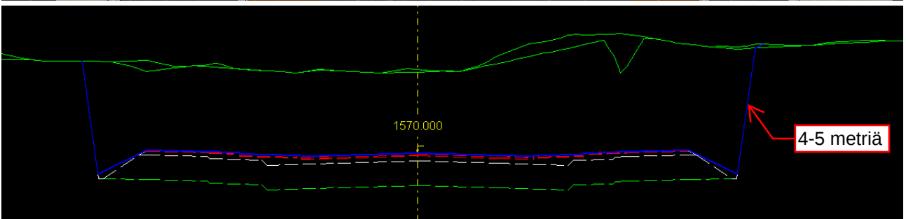
Mossin puistokadulla tonttien tasot jäämässä paikoin 4-5 metriä kadun pintaa ylempänä.
