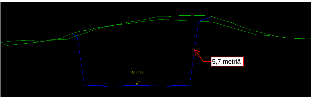
Bruuninkadulla katu leikkauksessa paikoin jopa 5,7 metriä
