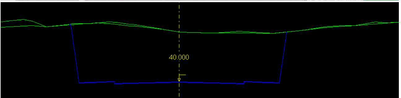
Bäckströminkujalla tontit n. 2,5 metriä kadun tasausta ylemmänä
