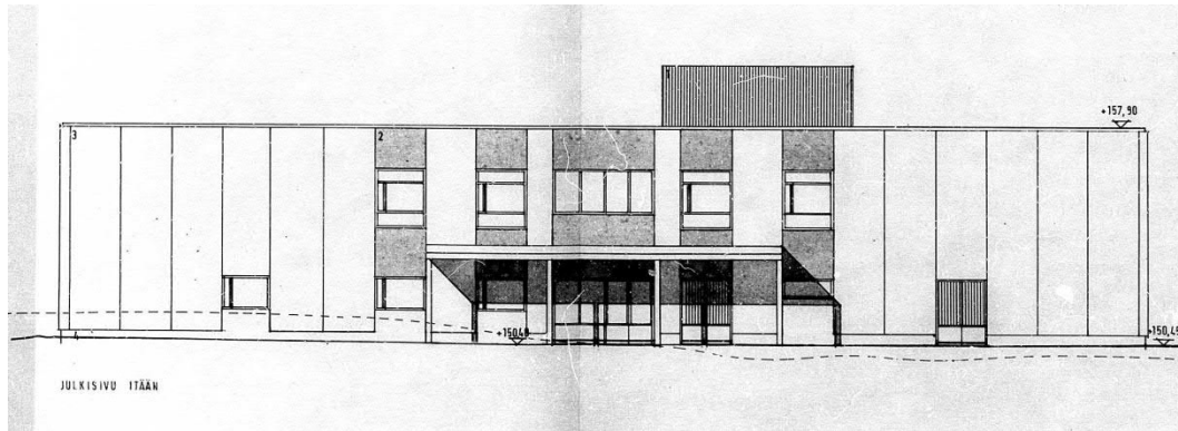
Kuva 6: Julkisivu itään
