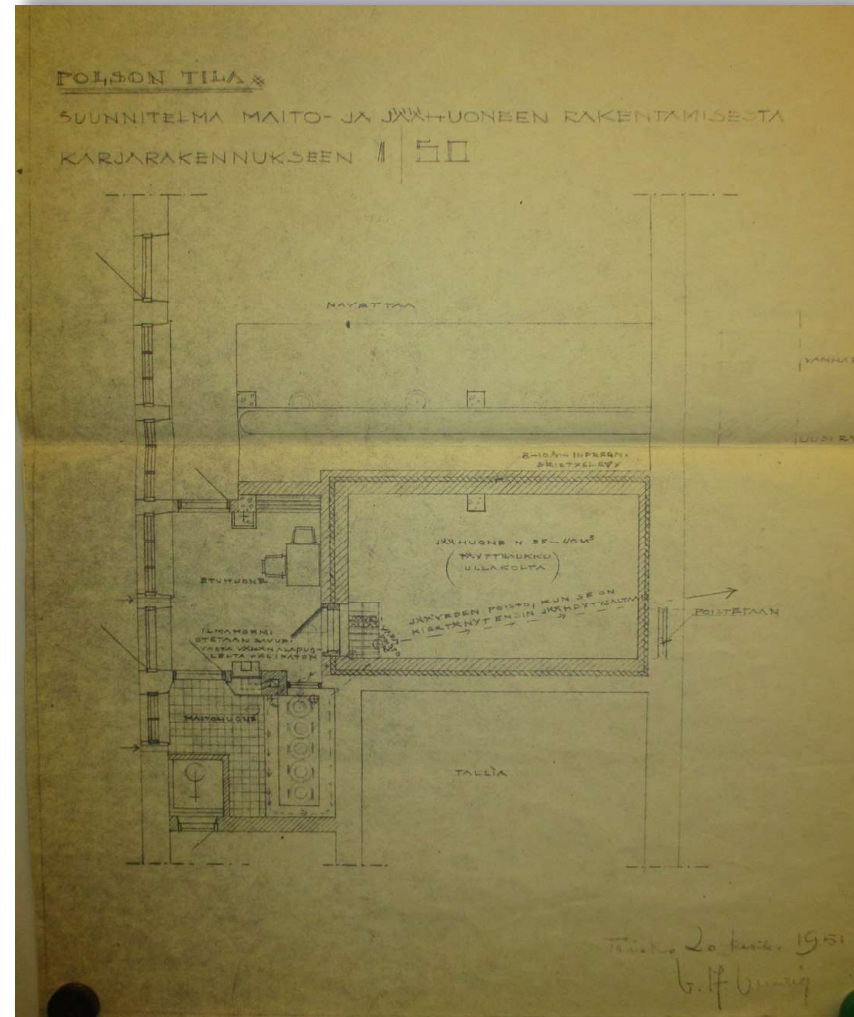
"Polson tila, Suunnitelma maito- ja jäähuoneen rakentamisesta karjarakennukseen". Pohjapiirrosote navetan ja tallin väliltä vuodelta 1951. Huoneet sijoittuivat lähelle rakennuksen kaakkoispäätä. Piirustuksen vasemmassa reunassa on rakennuksen lounaisjulkisivua. Maituhuone on viilennetty. Jäähuoneen täyttöluukku on ullakolla. (Lähde: Tipa)
