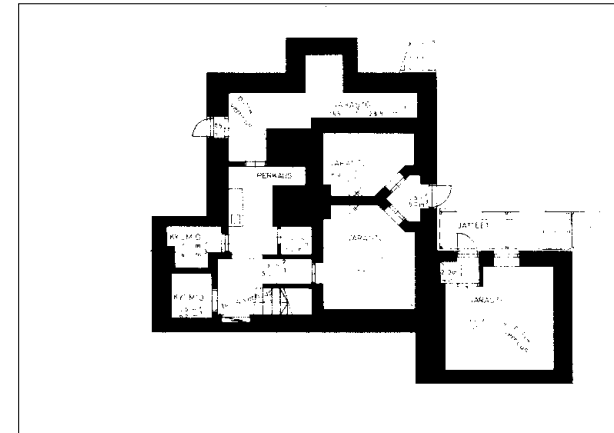
Kellarin pohjapiirros, 1976. (Rava) Tilat, joihin on yhteys vain ulkoa, ovat varastotiloja. Keittiöön portailla yhteydessä olevissa tiloissa ovat myös kylmiöt ja perkaustila.
