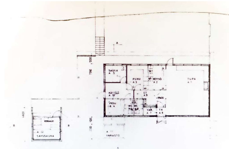
Arkkitehtitoimisto Antti Tähtisen saunasuunnitelmat saivat rakennusluvan 20.10.1976. (Lähde: Rava)
