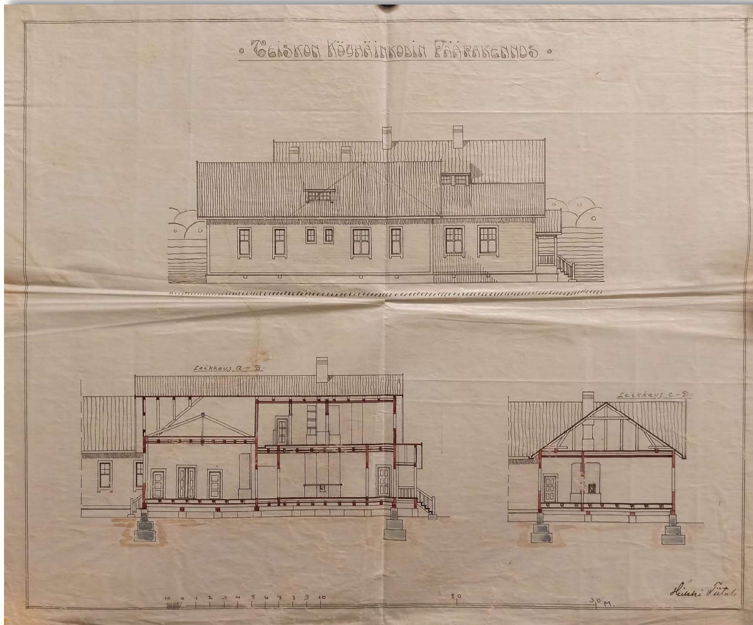
Heikki Tiitolan signeeraama julkisivu- ja leikkauspiirustus, oletettavasti vuodelta 1913. (Lähde: Tipa)
