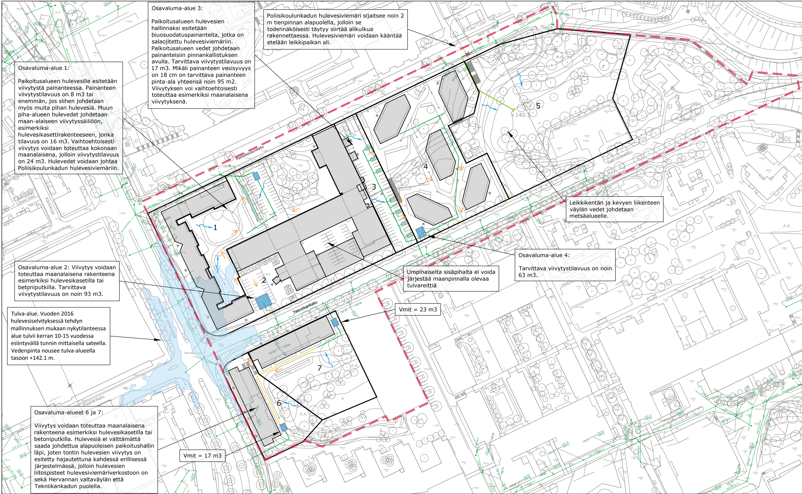
ASEMAKAAVAN 8772 HULEVESISELVITYS Liite 1: Hulevesien hallinnan yleissuunnitelma 1:1500 (A3) Päivitys 20.6.2021 SKI
