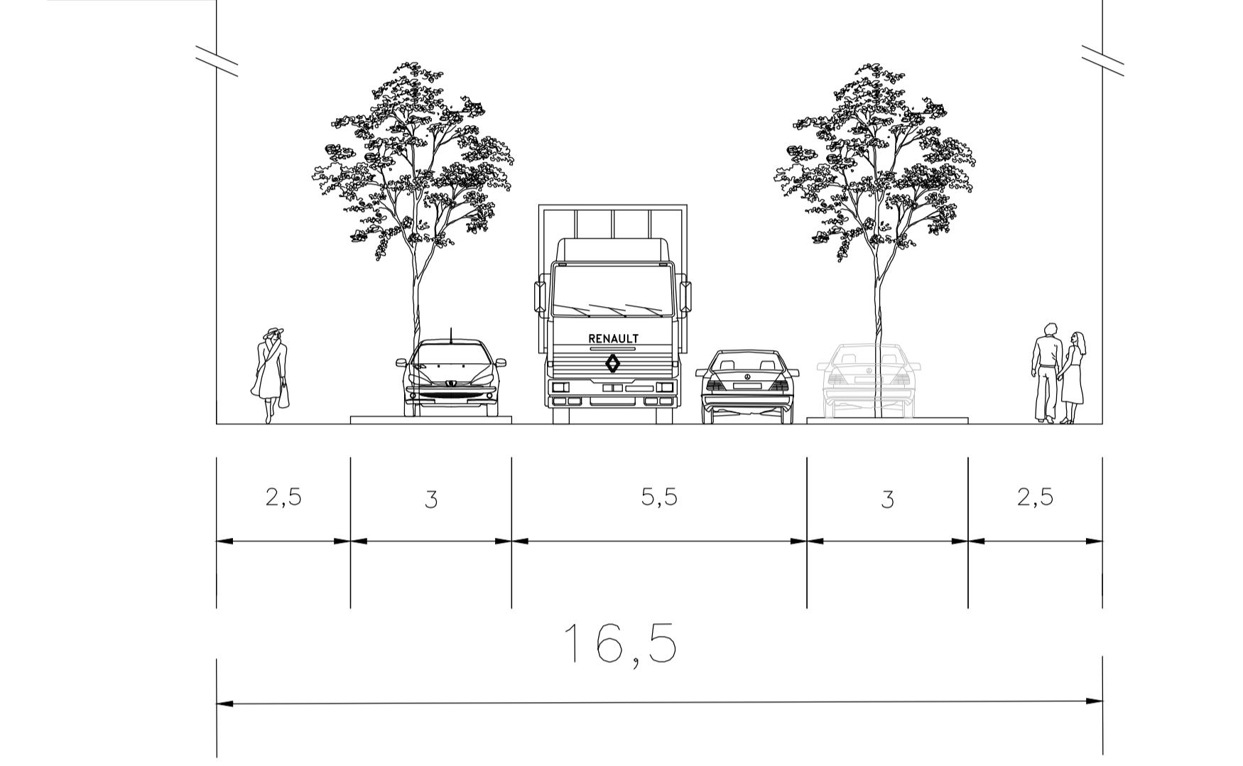
Leikkaus B-B, Kuivaamonkatu
