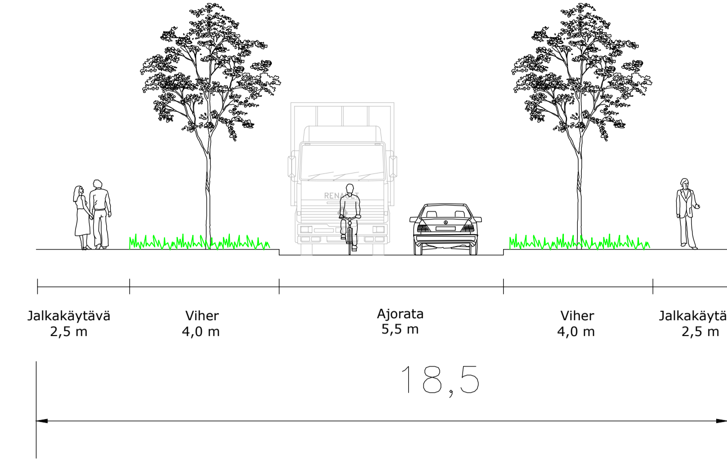
Leikkaus D-D, Tehdaskartanonkatu
