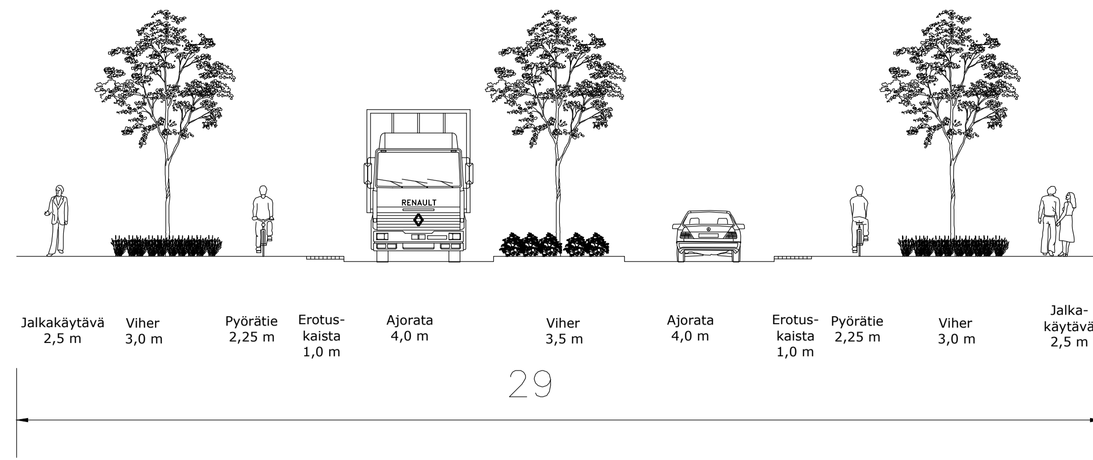
Leikkaus E-E, Tehdaskartanonkatu
