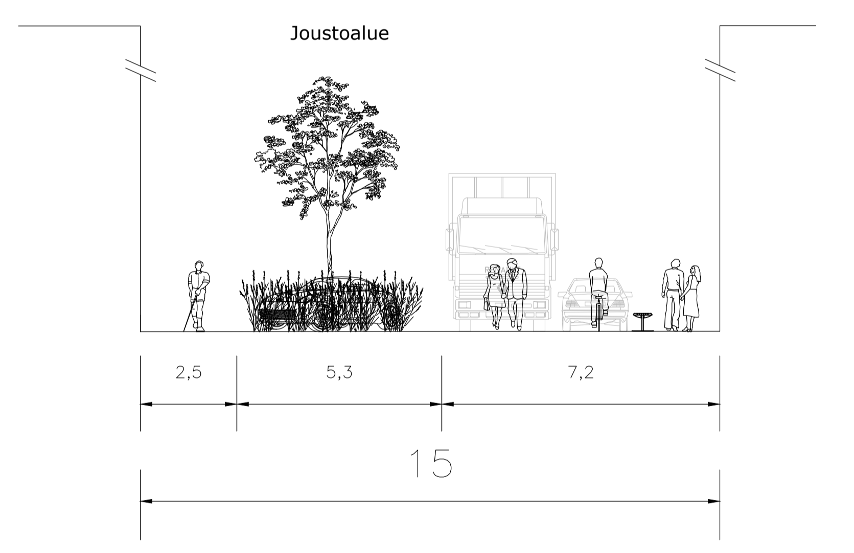
Leikkaus B-B, Kuivaamonkatu
