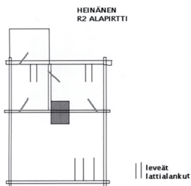
Pirtin pohjakaavio. KN 2007
