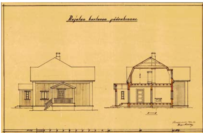
Birger Federleyn piirustuksia päärakennuksesta. (Eeva Leino)
