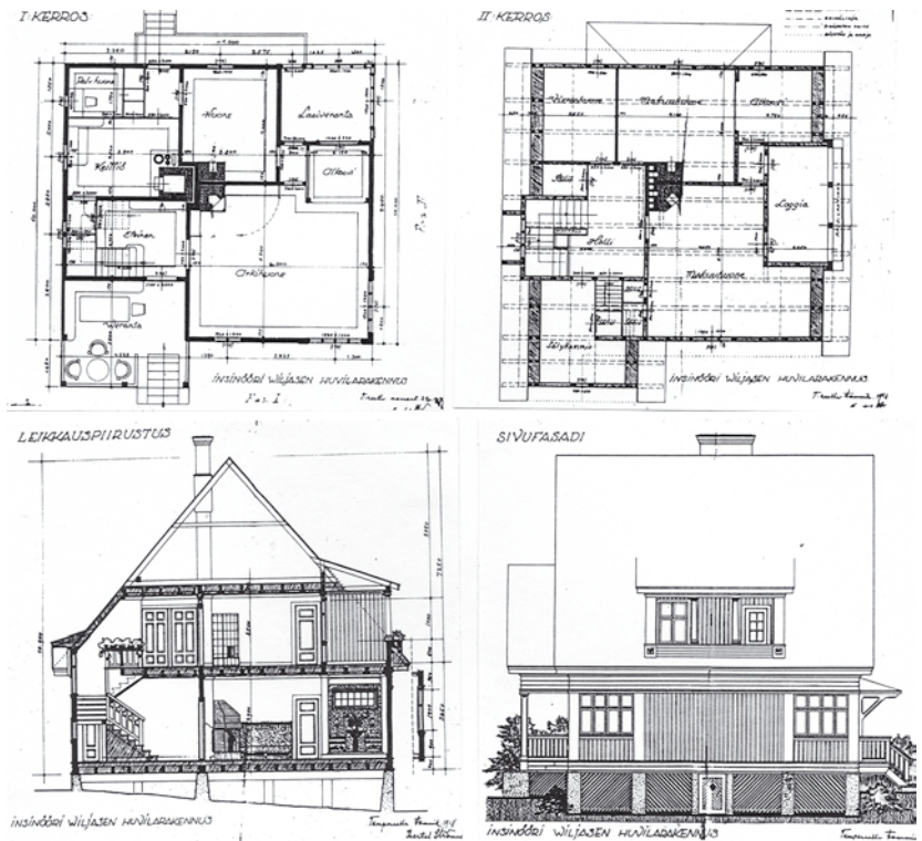
Nuoren Bertel Strömmerin piirustukset vuodelta 1918. TKA
