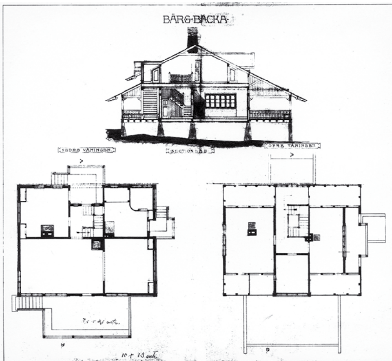
Frithiof Strandellin piirustukset. TKA
