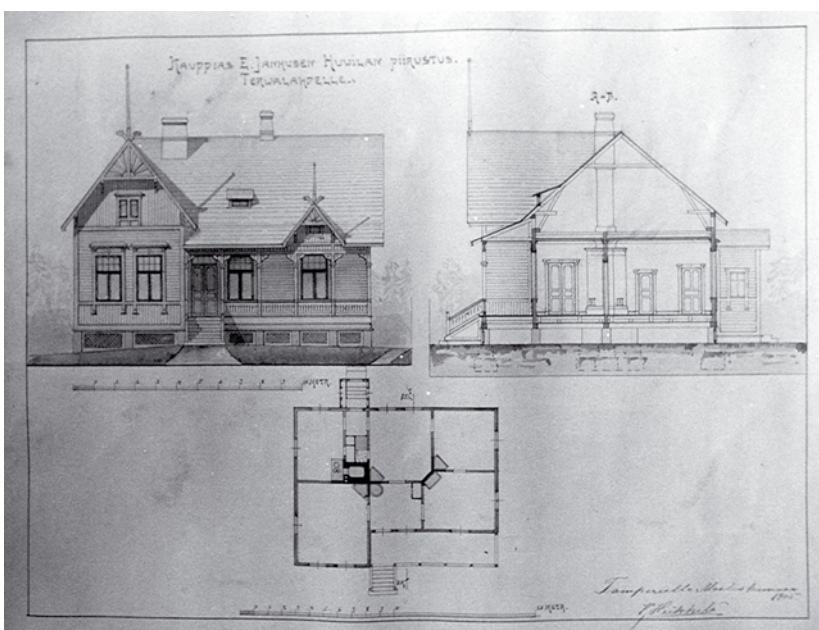
Vihtori Heikkilän piirustukset vuodelta 1905. TKA
