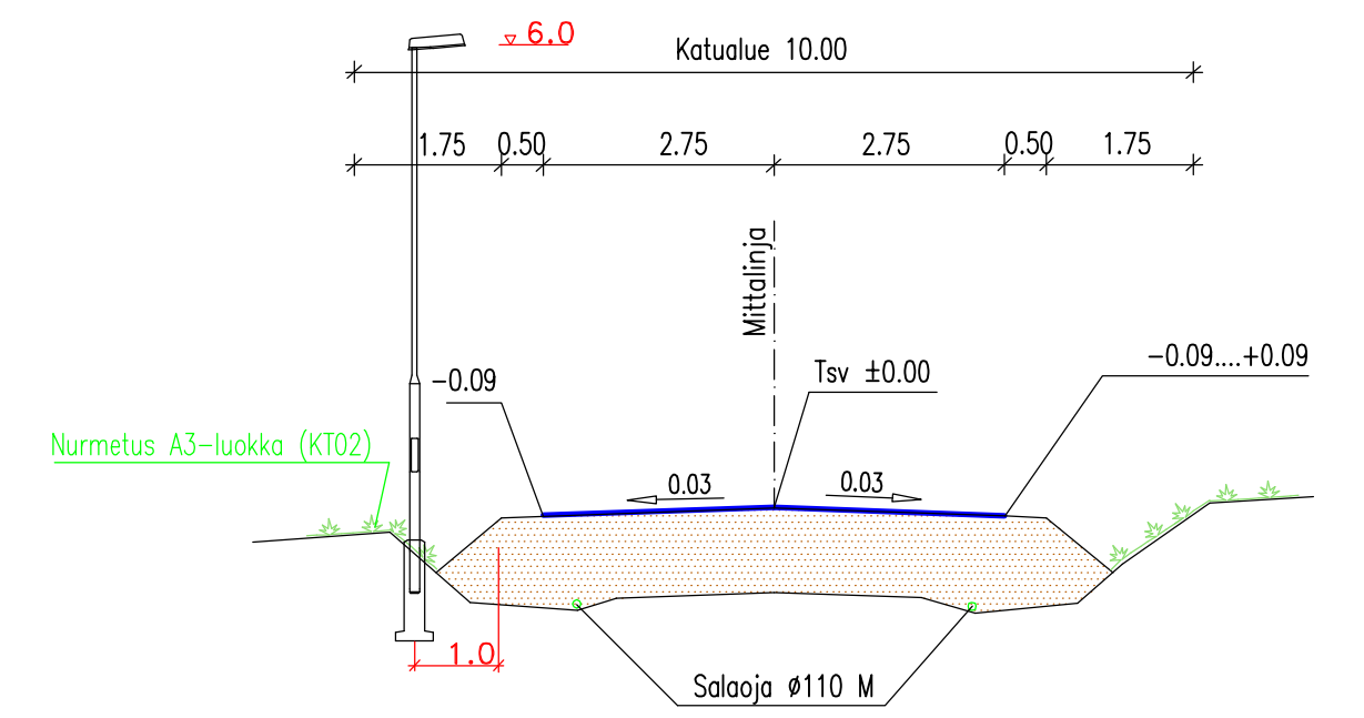
TYYPPIPOIKKILEIKKAUS 1:100
